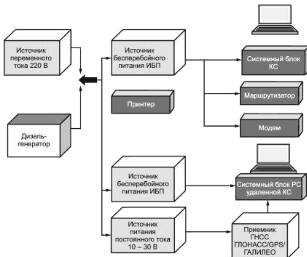
Рисунок 4 — Типовая схема электропитания аппаратуры УКУС
