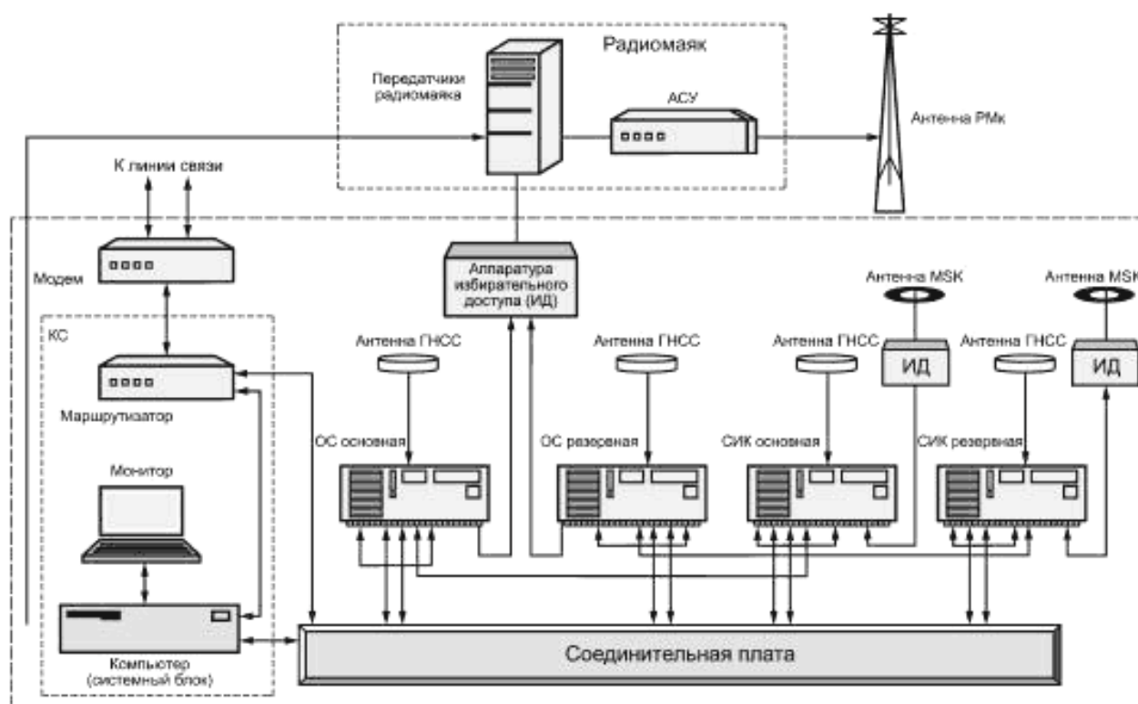
Рисунок 1 — Контрольно-корректирующая станция ГНСС ГЛОНАСС/GPS/ГАЛИЛЕО
