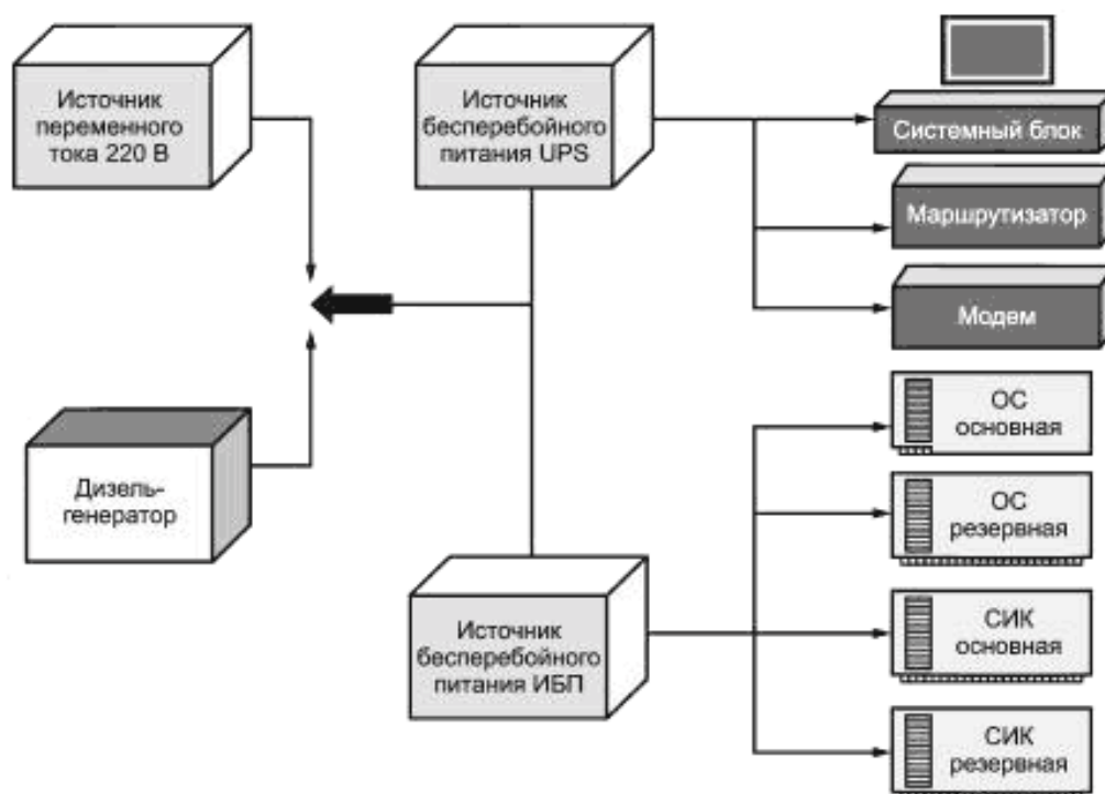
Рисунок 2 — Схема электропитания аппаратуры ККС
