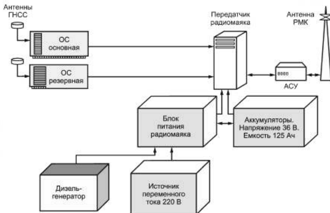
Рисунок 3 — Схема межблочных соединений и питания радиомаяка
