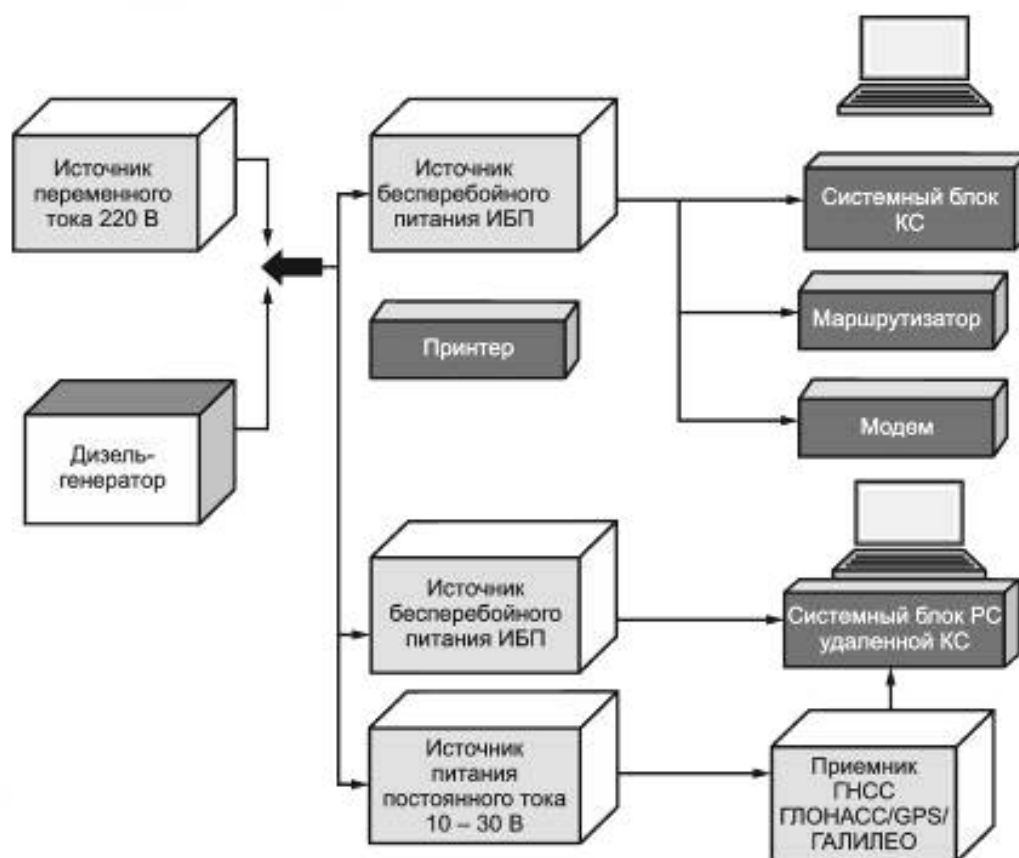
Рисунок 4 — Типовая схема электропитания аппаратуры УКУС
