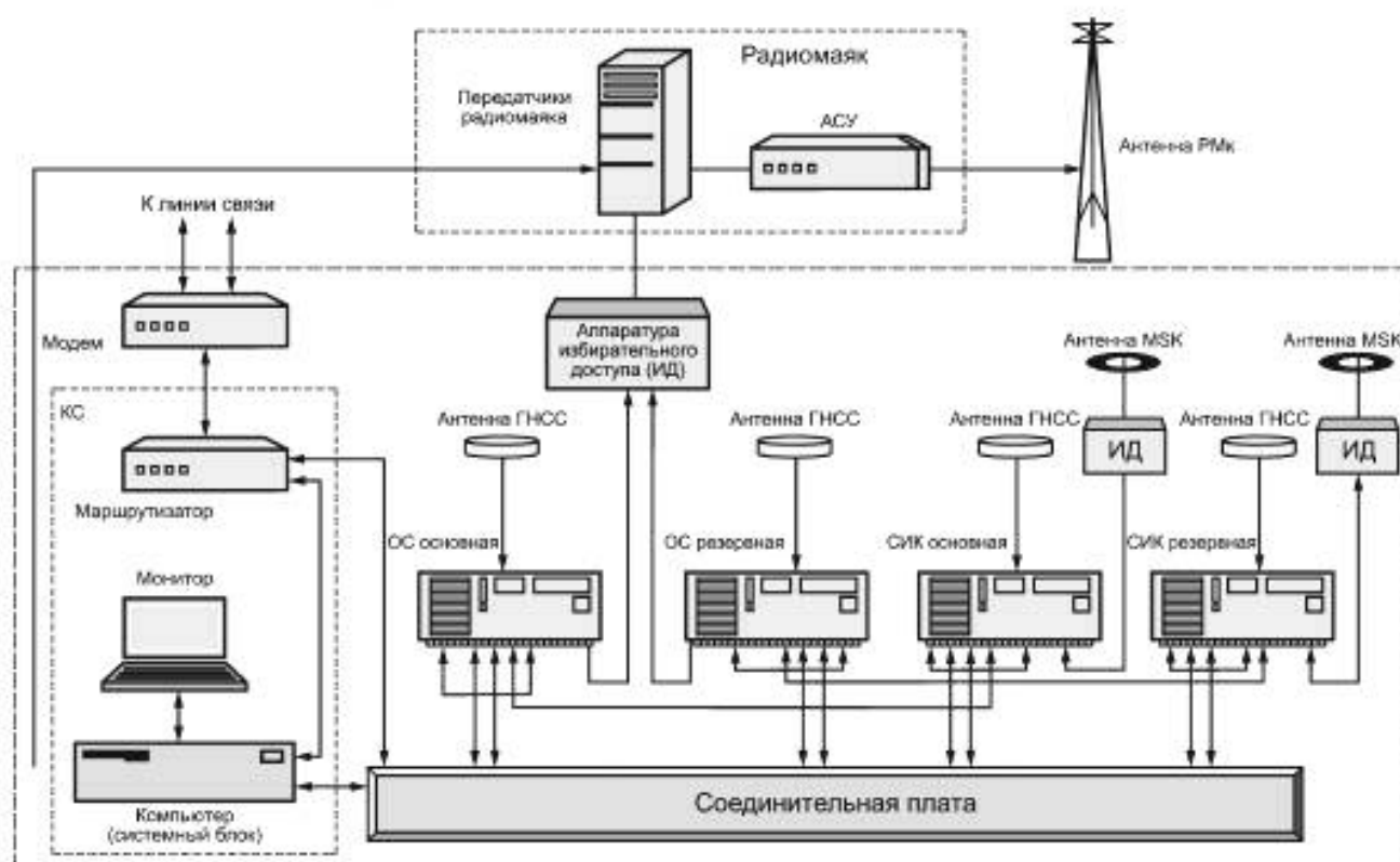
Рисунок 1 — Контрольно-корректирующая станция ГНСС ГЛОНАСС/GPS/ГАЛИЛЕО
