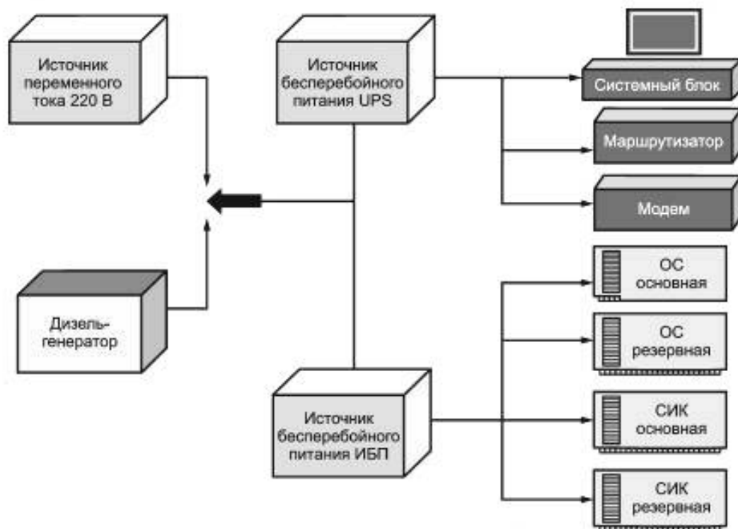
Рисунок 2 — Схема электропитания аппаратуры ККС
