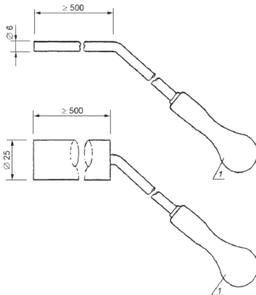
Рисунок А.1 — Конструкция щупов
