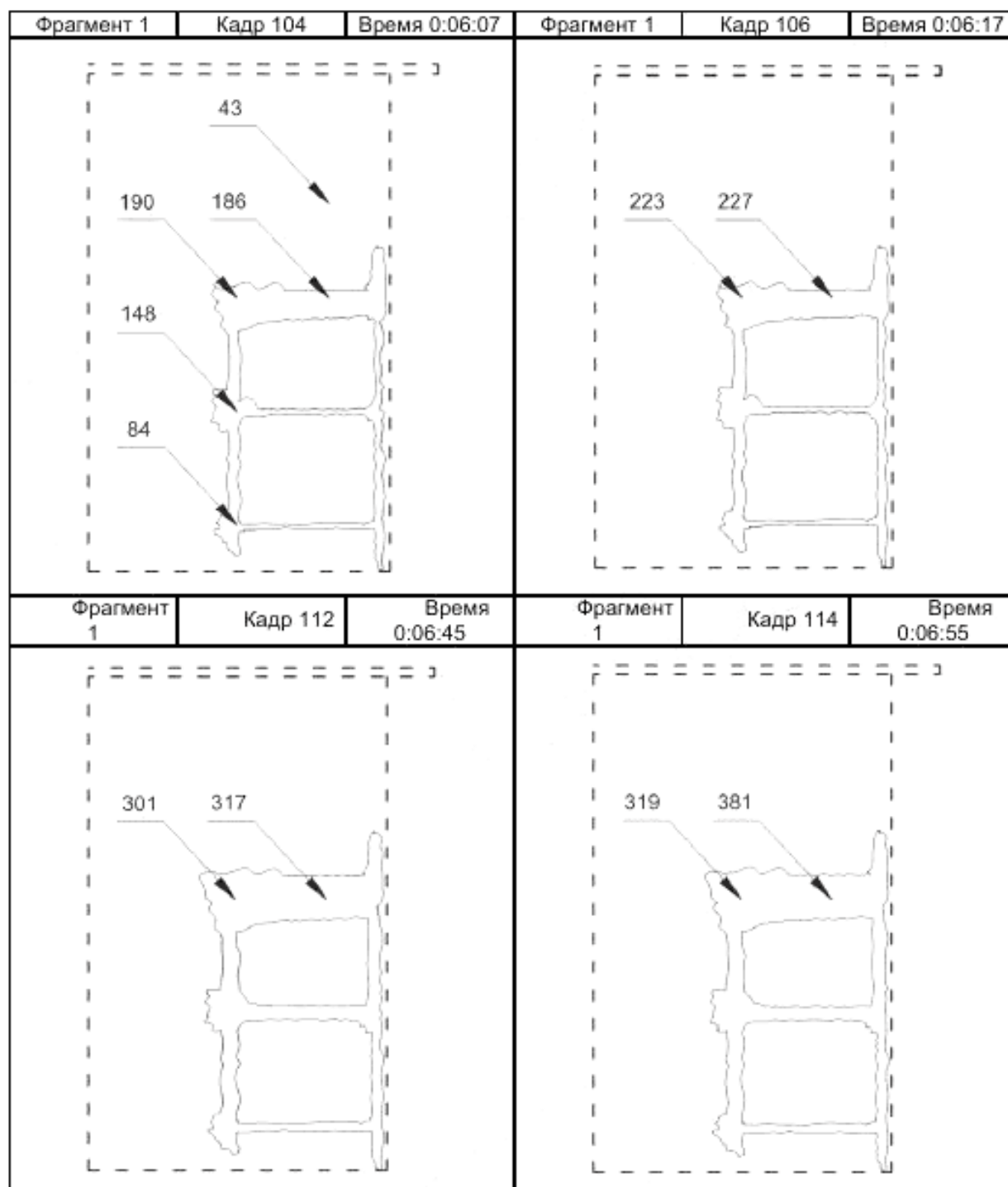
Рисунок Ж.4 — Пример оформления обзорных термограмм
