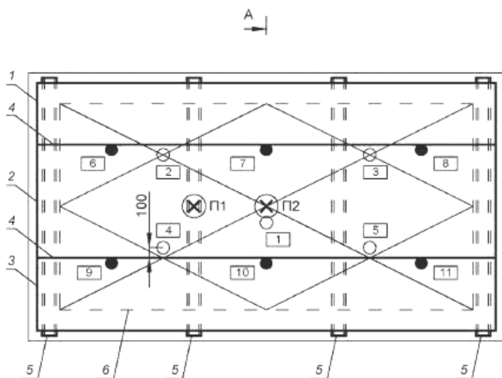
а — продольный разрез и вид сверху Рисунок Б.3, лист 1
