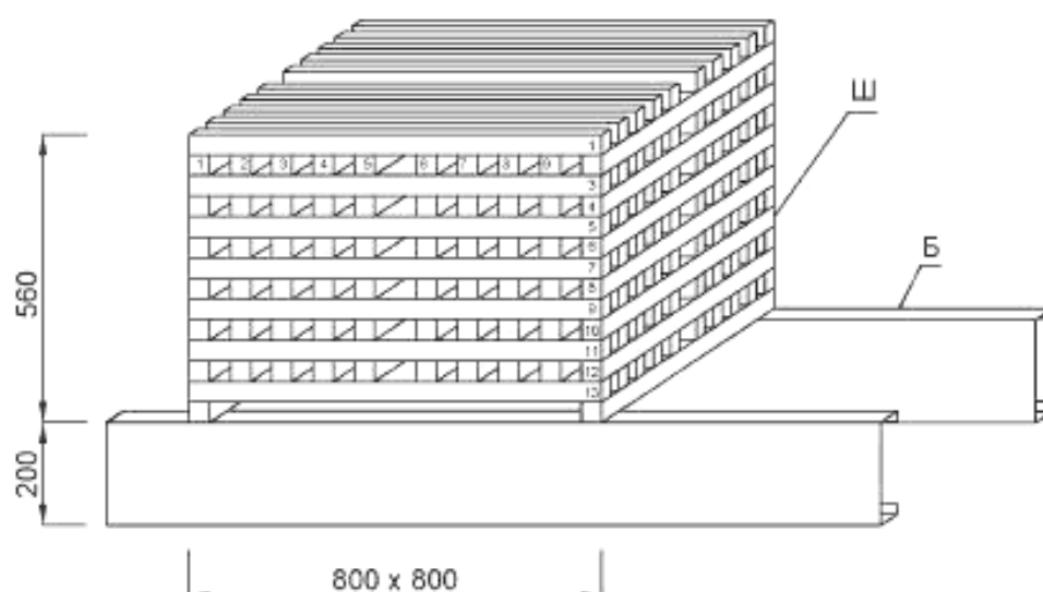
Ш – штабель из брусков размером 40×40×800 мм; Б – балки каркаса
