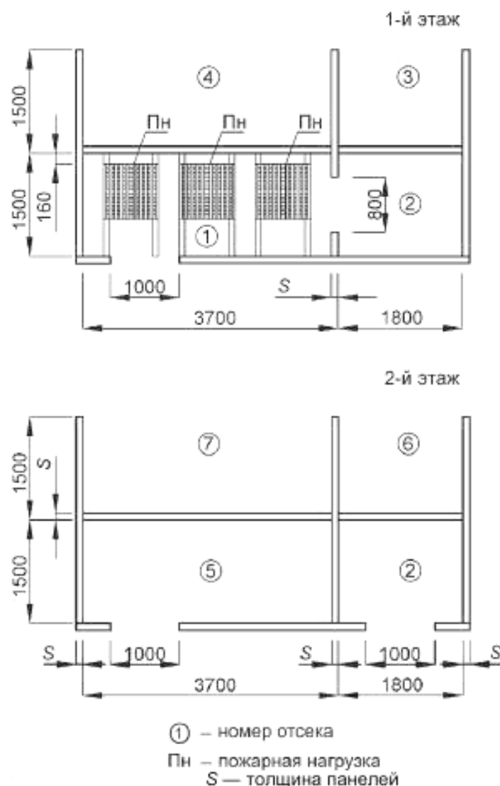
Рисунок Г.4 – Поэтажные планы
