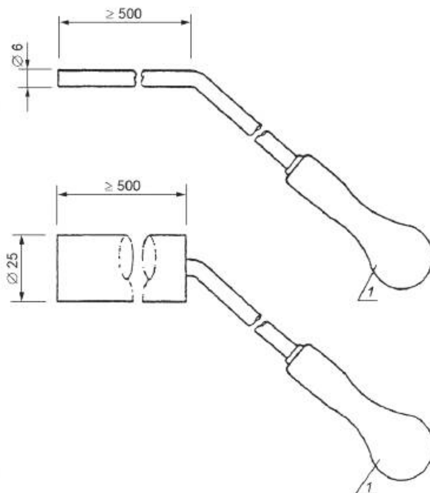
Рисунок А.1 — Конструкция щупов
