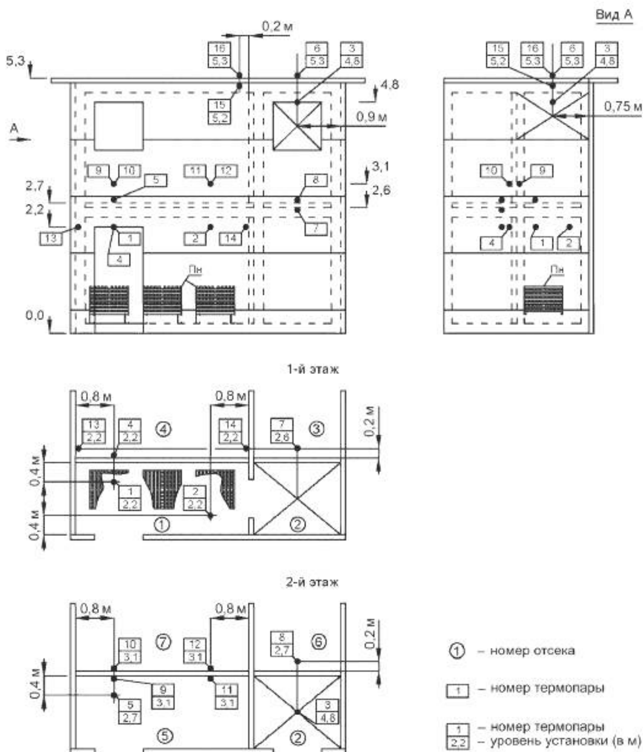
Рисунок Г.5 — Схема расстановки термодатчиков. Уровни установки 3,1 и 5,3 м указаны для панелей толщиной 100 мм и должны изменяться на разницу между фактической толщиной и указанным значением
