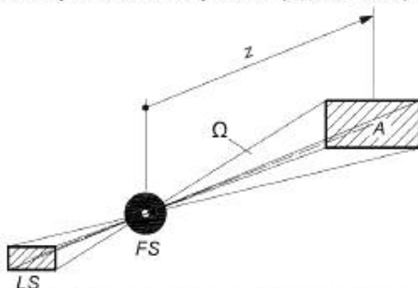
FS — первая апертура площадью a ; \Omega — телесный угол излучения источника света LS; A — площадь второй апертуры; z — расстояние между первой апертурой FS и второй апертурой площадью A
