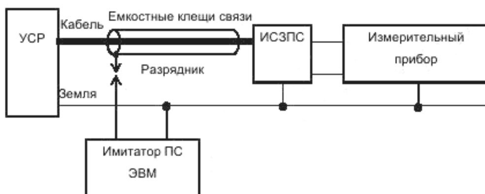
е) СЗПС-СЭП-6, СЗПС-ПЛС-3, режим холостого хода с использованием емкостных клещей.
