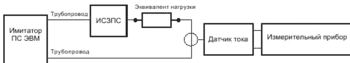
а) стандартных параметров СЗПС-МК-1...3 (на эквивалент нагрузки);
