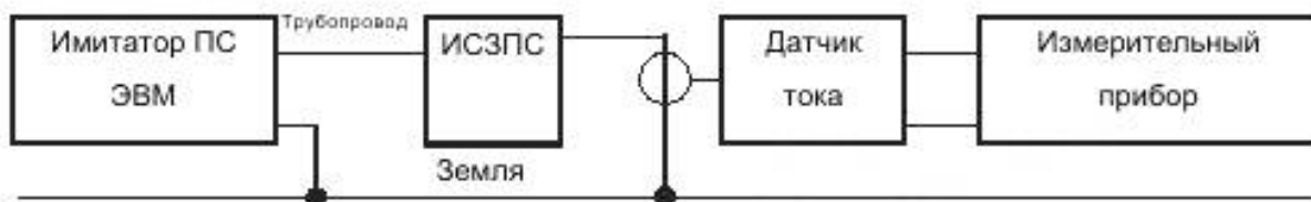
д) СЗПС-МК, режим короткого замыкания, цепь "трубопровод или иная металлоконструкция-земля";
