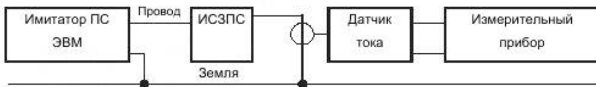
г) СЗПС-СЭП, СЗПС-ПЛС, режим короткого замыкания, цепь "провод-земля";
