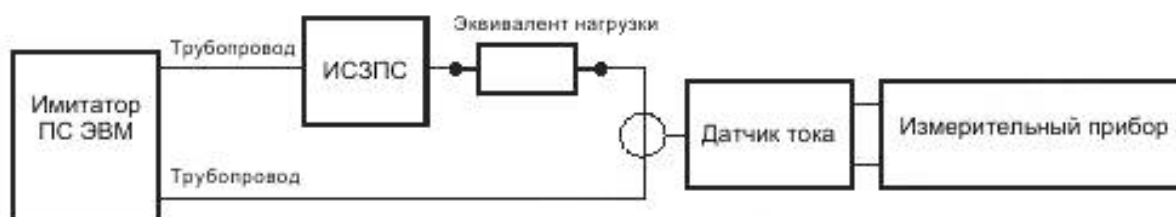
а) стандартных параметров СЗПС-МК-1...3 (на эквивалент нагрузки);
