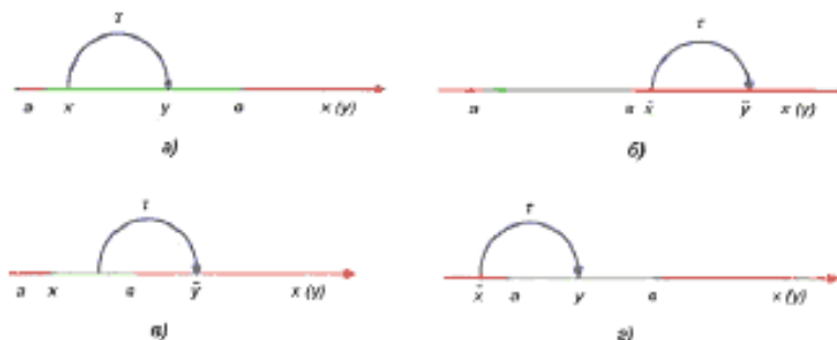
Рисунок 1 Случаи возникновения ошибок I и II рода при измерениях
