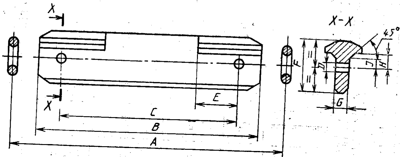
Рисунок 1 — Размеры Т-образных скребков
