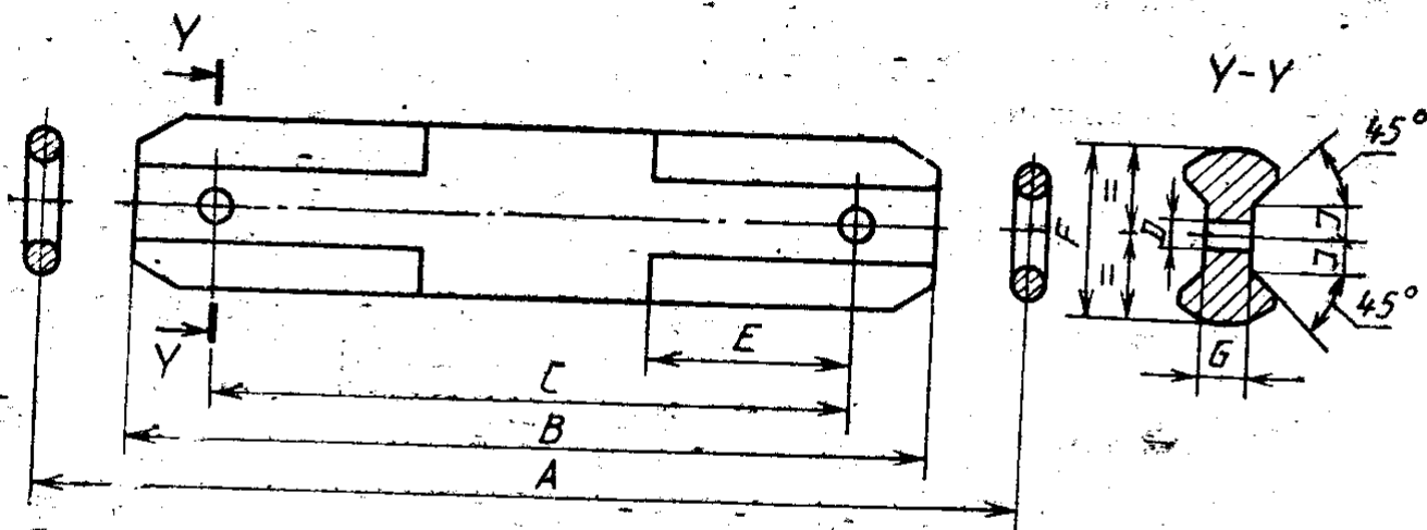
Рисунок 2 — Размеры I-образных скребков
