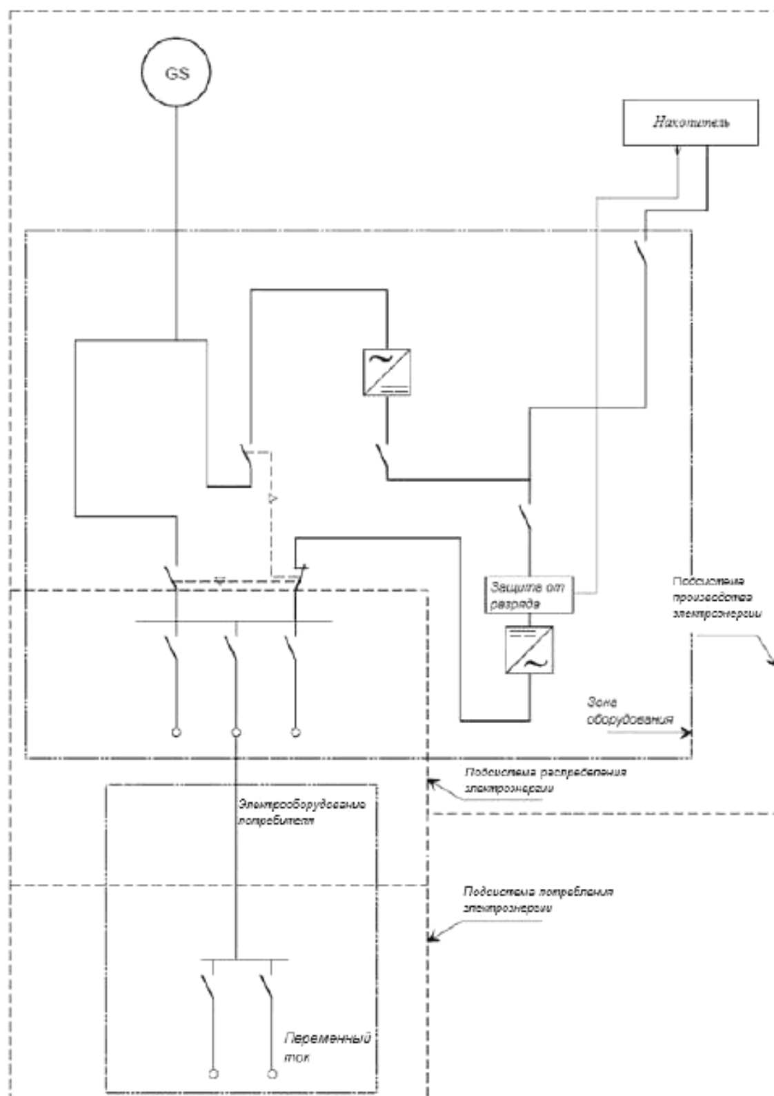
Рисунок Д.18 – Система типа Т 6 С
