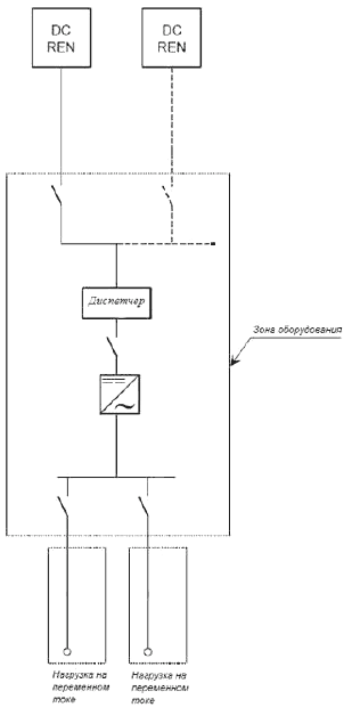
Рисунок Д.3 – Система типа T 1I -с
