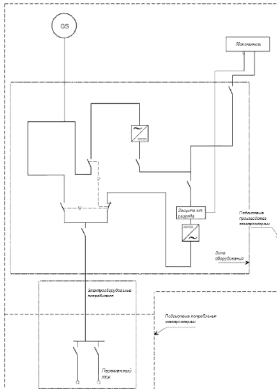
Рисунок Д.10 – Система типа Т 6 I
