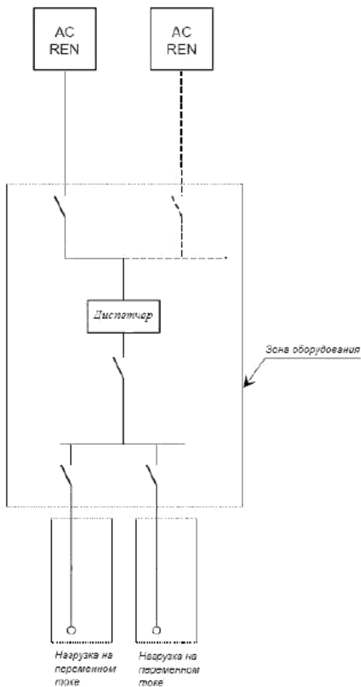
Рисунок Д.2 – Система типа T 1 I-b
