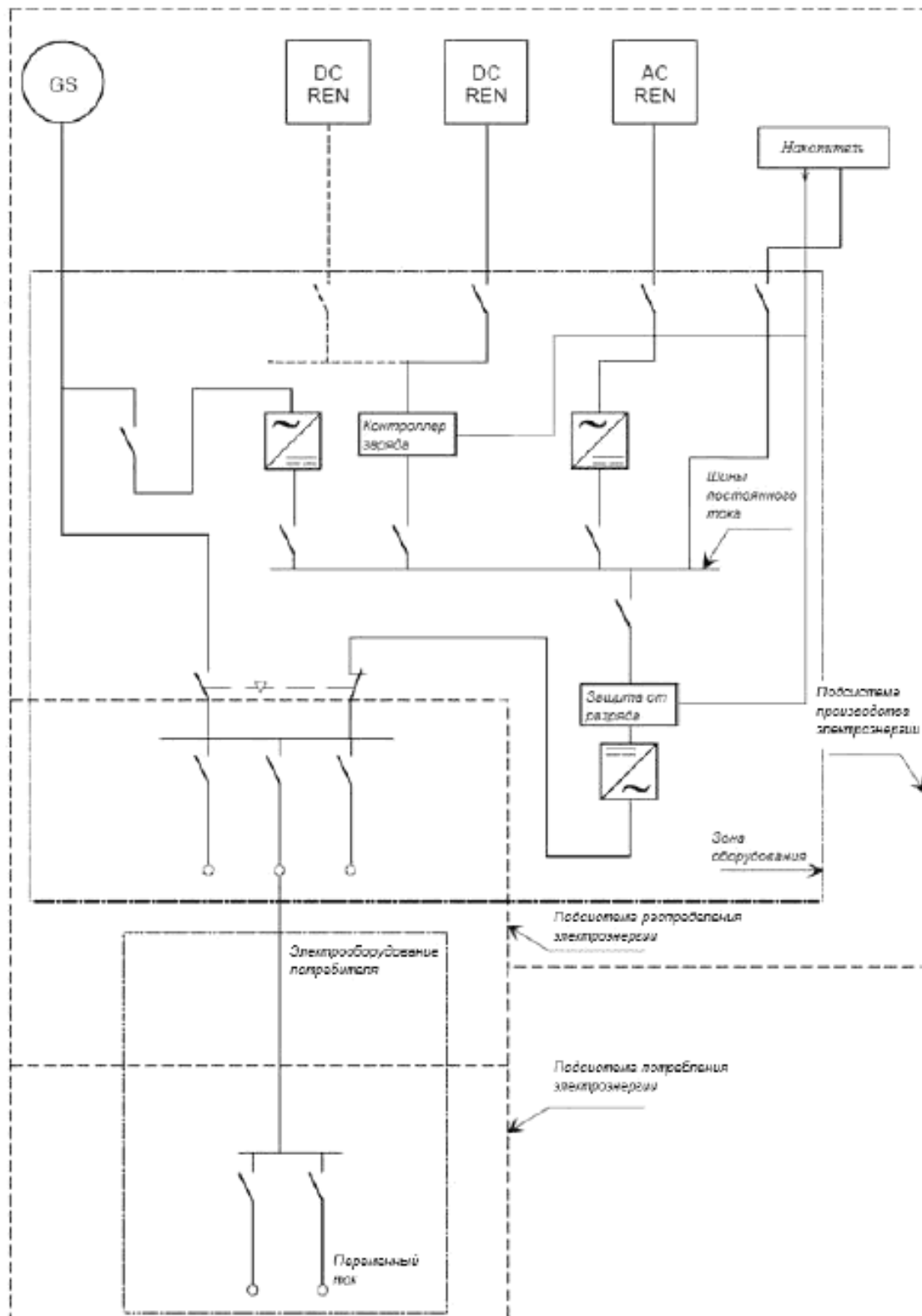
Рисунок Д.15 – Система типа Т 4 С-а
