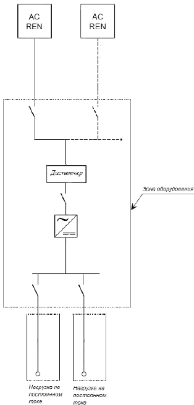
Рисунок Д.4 – Система типа T 1 I-d.
