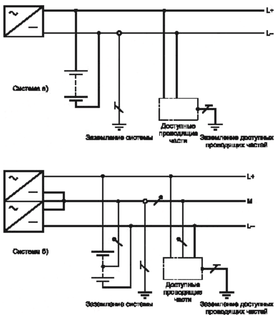
Рисунок Б.8 — ТТ система постоянного тока
