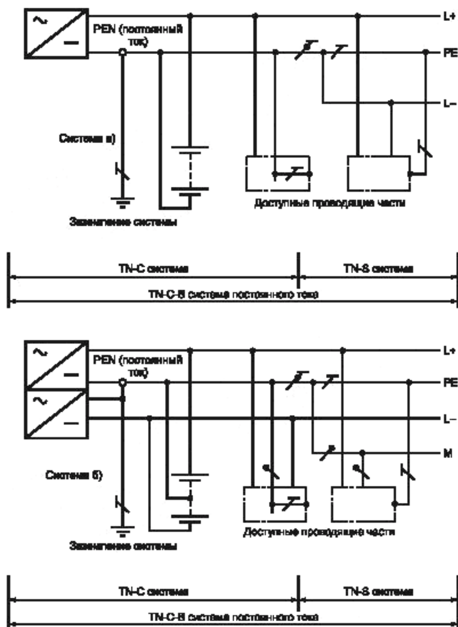
Рисунок Б.7 — TN-C-S система постоянного тока
