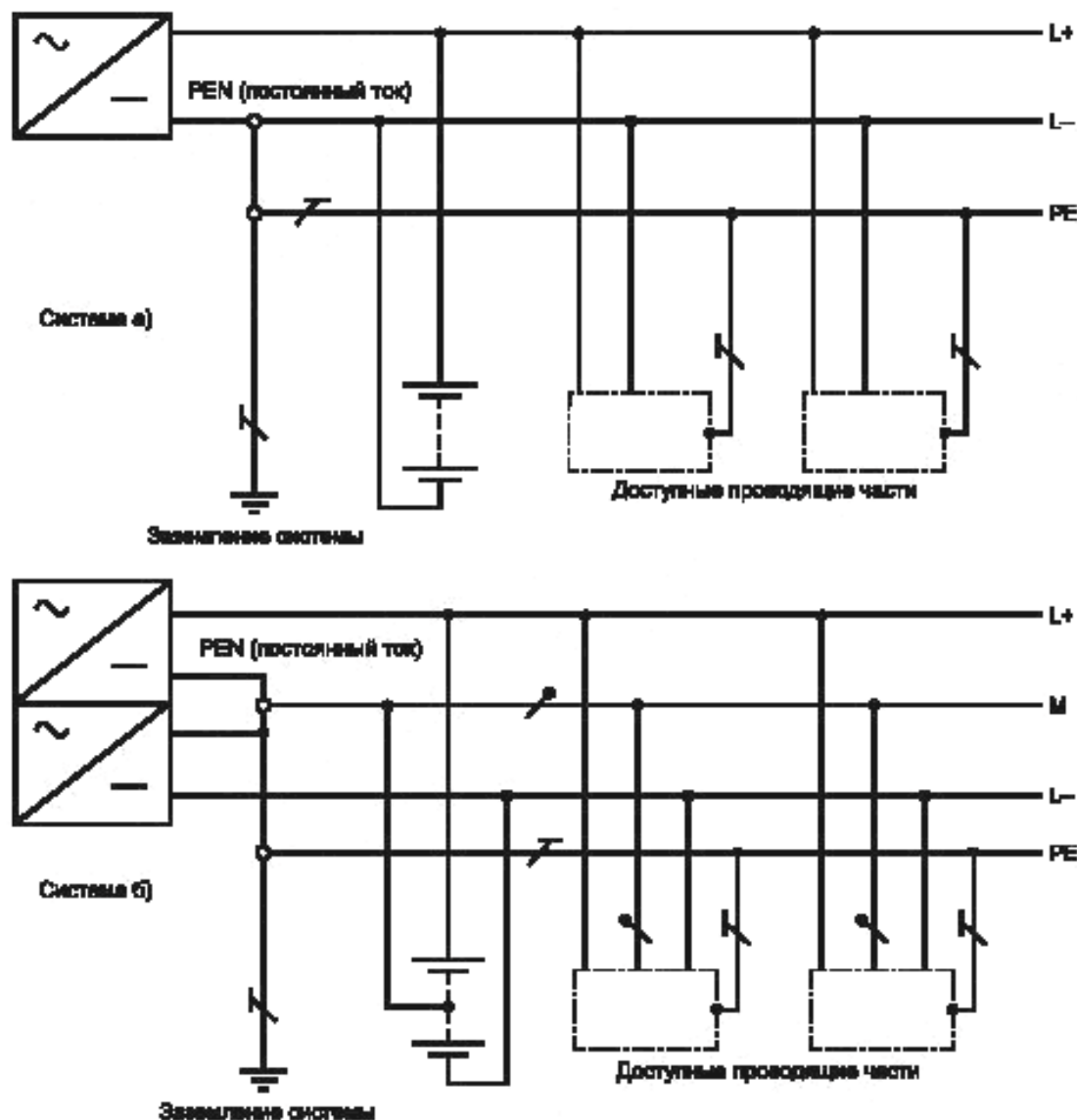
Рисунок Б.5 — TN-S система постоянного тока
