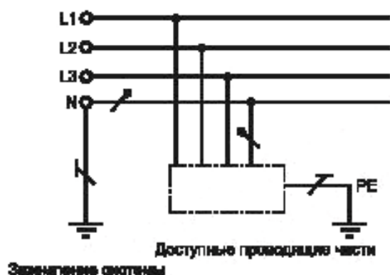
Рисунок Б.4 — TT система
