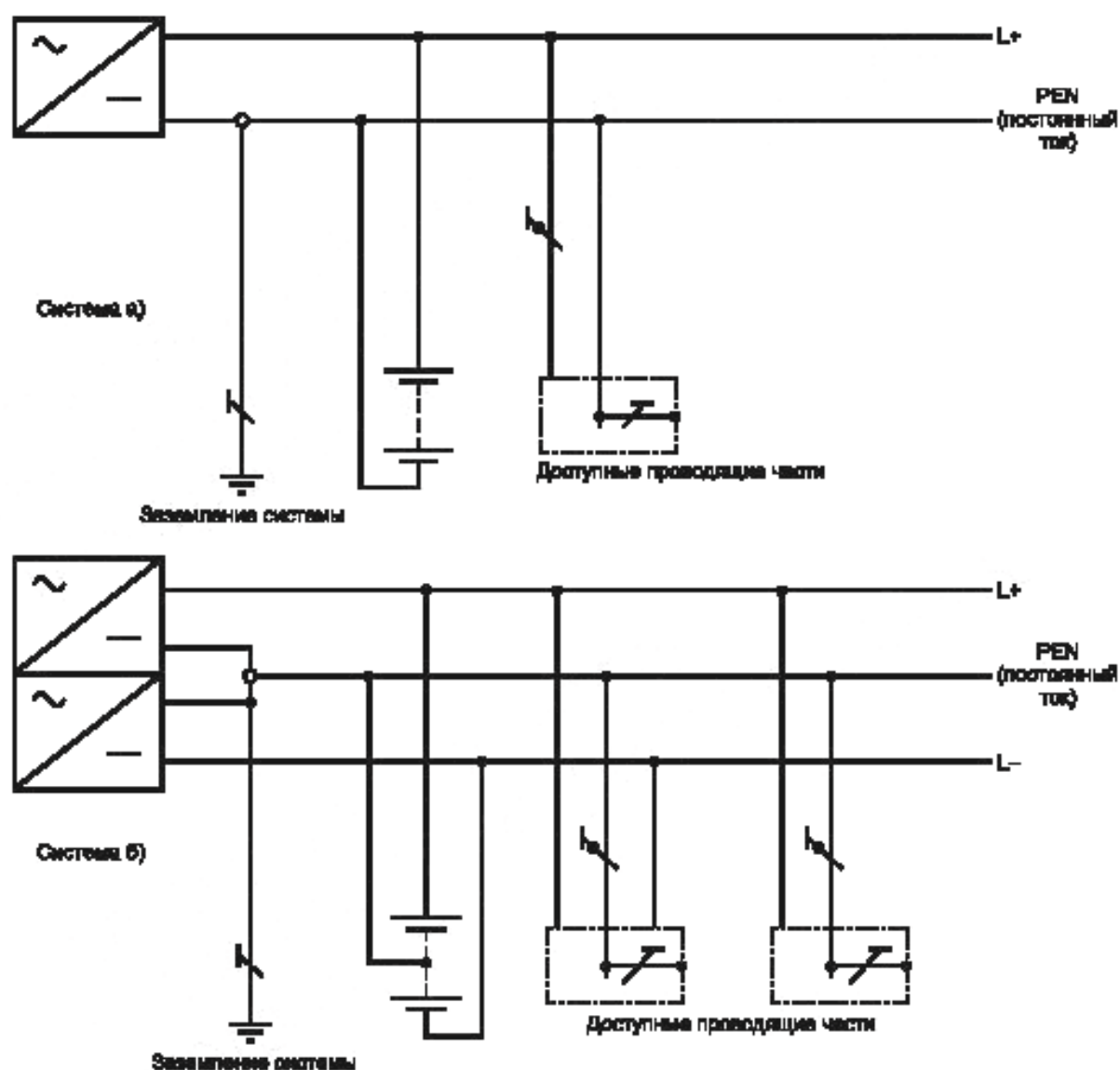
Рисунок Б.6 — TN-C система постоянного тока
