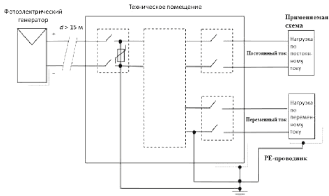
Рисунок 5 — Конфигурация H — только солнечная фотозлектрическая батарея индивидуальной системы электроснабжения P < 500 \text{ Вт} — с инвертором — d > 15 \text{ м}
