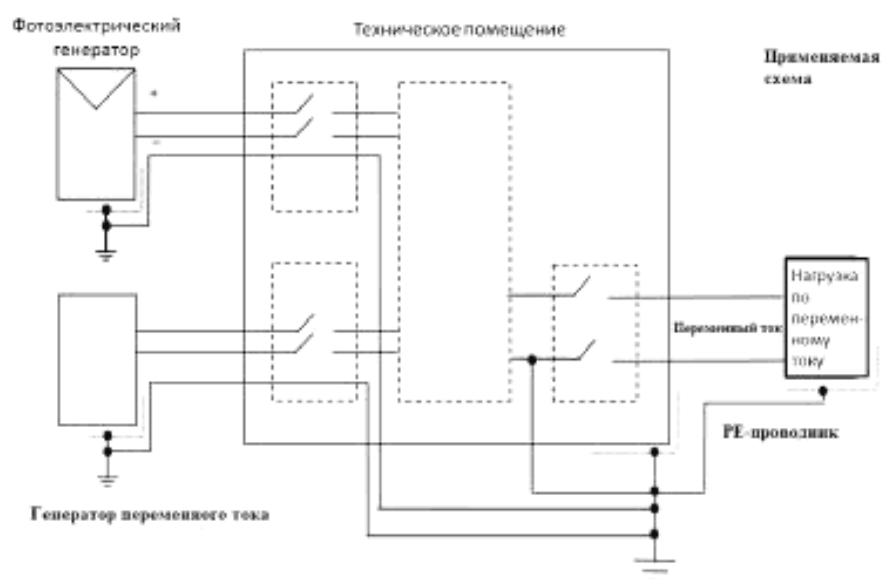
Рисунок 7 — Конфигурации I и K — только солнечная фотоэлектрическая батарея индивидуальной или коллективной систем электроснабжения P < 500 Вт — с инвертором — d > 15 м
