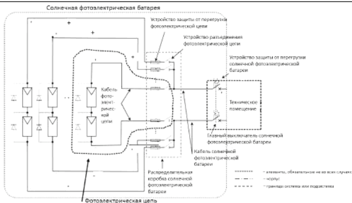
Рисунок 11 — Схема солнечной фотоэлектрической батареи — случай мультицепи
