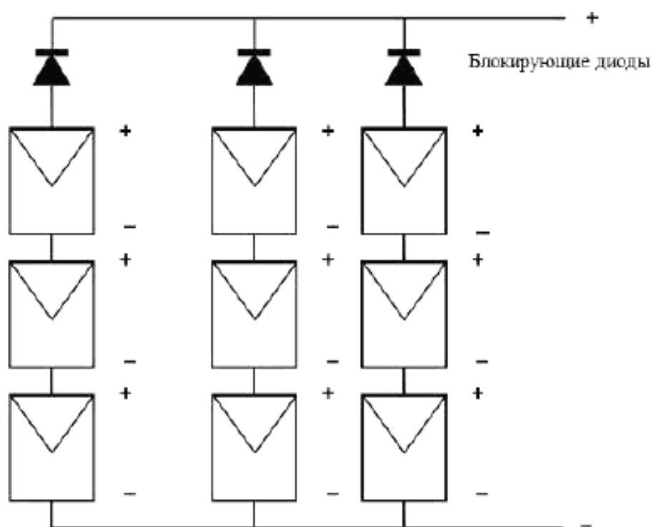
Рисунок 14 — Исполнение блокирующего диода (пример)
