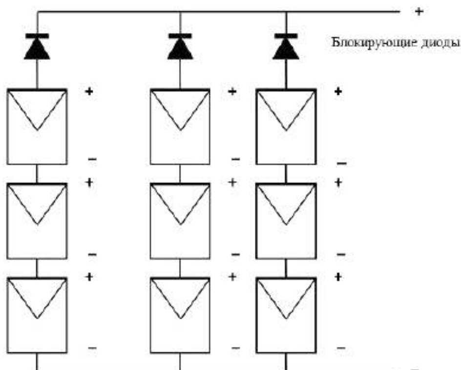
Рисунок 14 — Исполнение блокирующего диода (пример)
