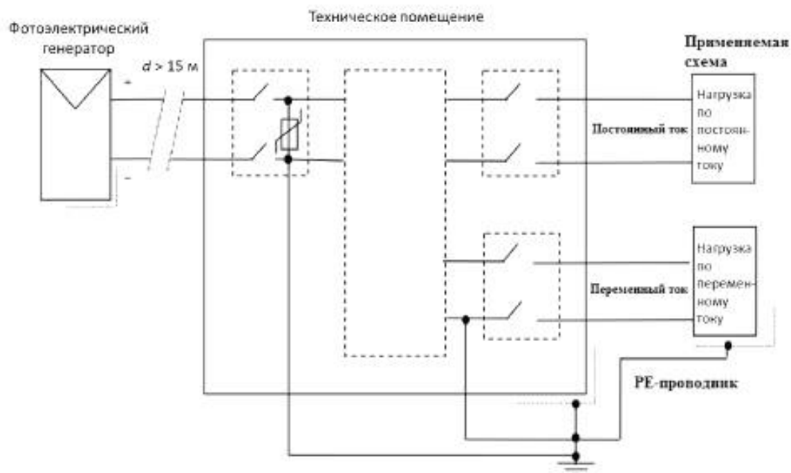
Рисунок 5 — Конфигурация Н — только солнечная фотоэлектрическая батарея индивидуальной системы электроснабжения P < 500 \text{ Вт} — с инвертором — d > 15 \text{ м}
