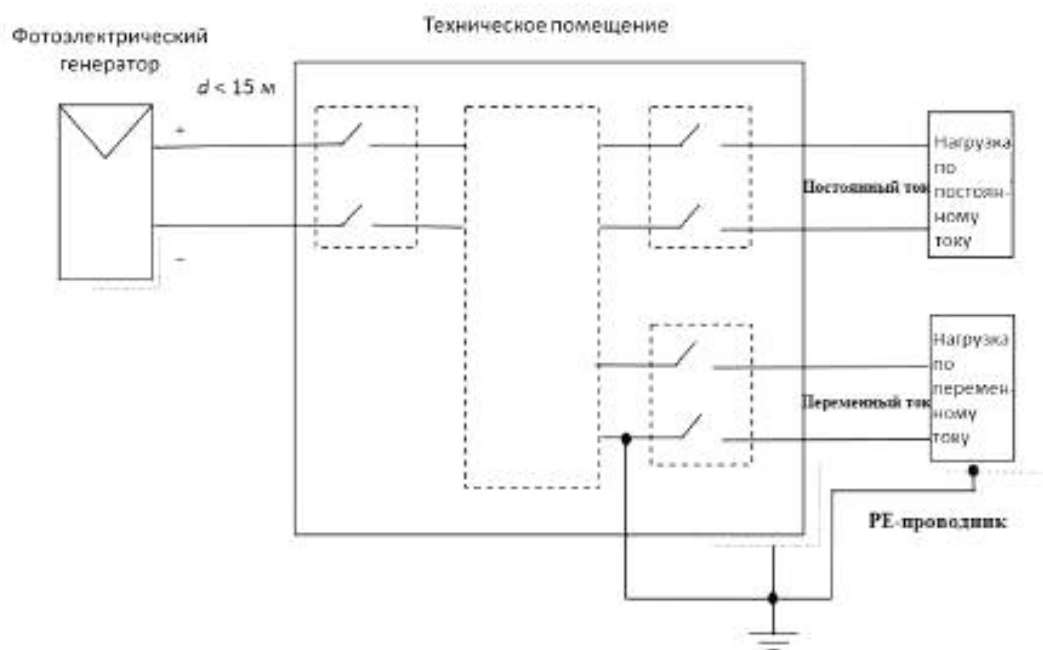
Рисунок 3 — Конфигурация G — только солнечная фотозлектрическая батарея индивидуальной системы электроснабжения P < 500 \text{ Вт} — без инвертора — d > 15 \text{ м}
