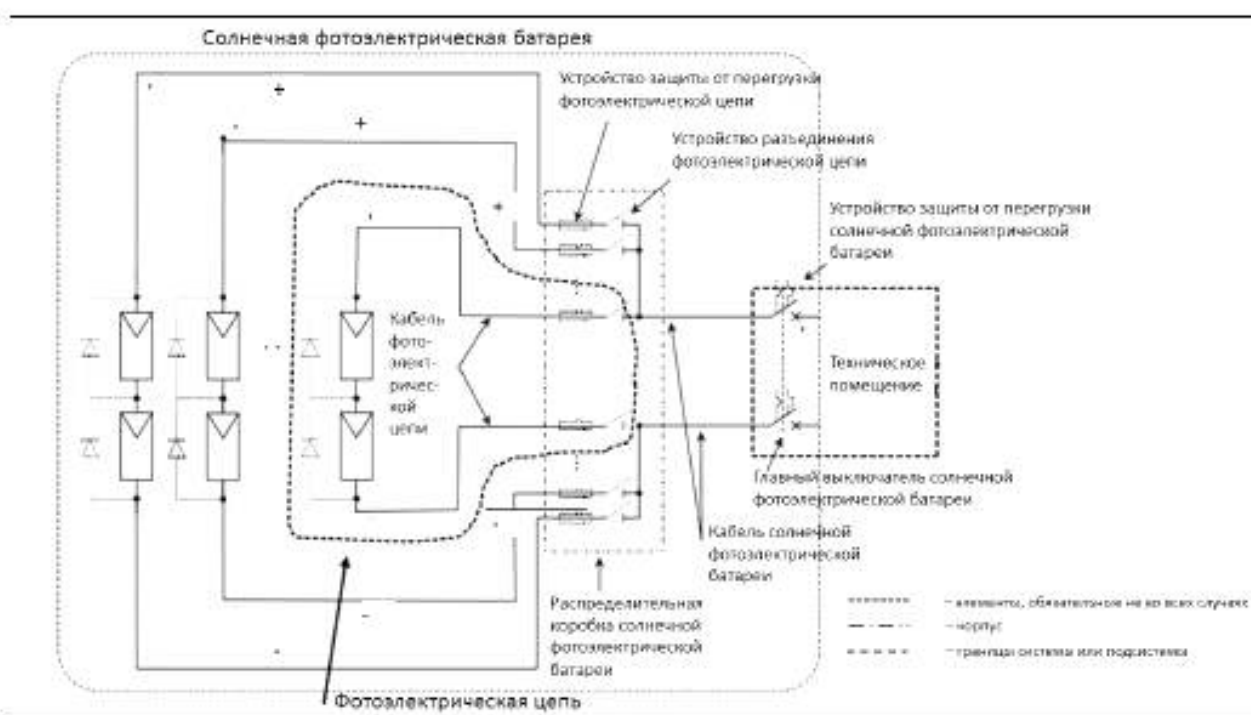
Рисунок 11 — Схема солнечной фотоэлектрической батареи — случай мультицепи
