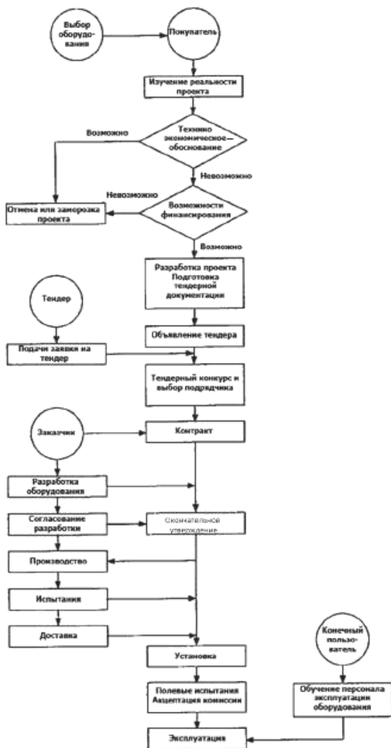
Рисунок ДА.1 – Блок-схема процедуры создания гидроэлектростанции
