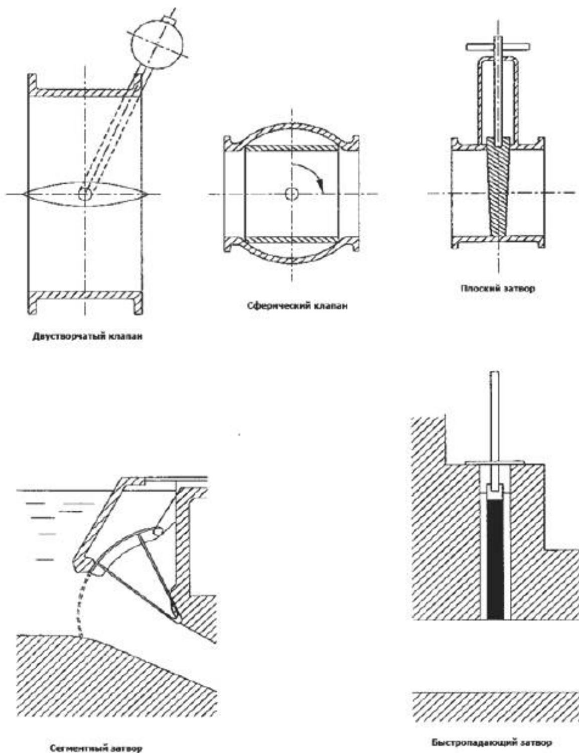
Рисунок ДА.7 –Примеры затворов
