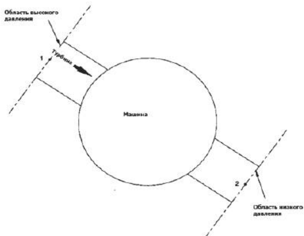
Рисунок ДА.8 – Принципиальная схема работы гидромашины
