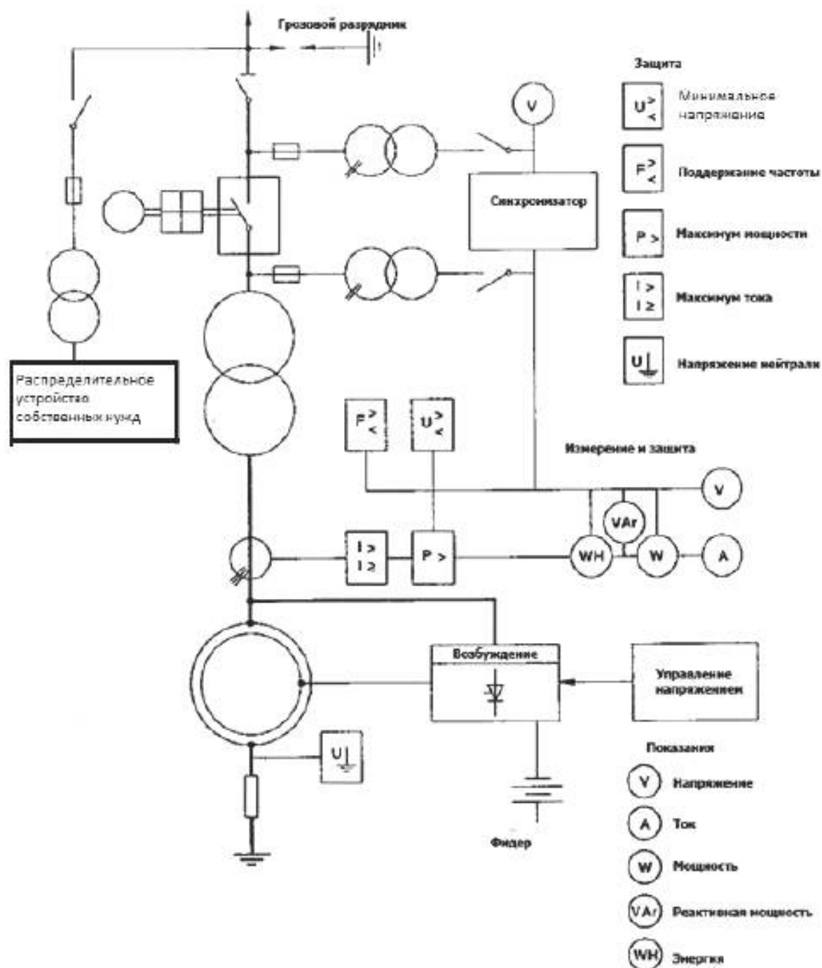
Рисунок ДА.66 – Однолинейная схема – Синхронный генератор
