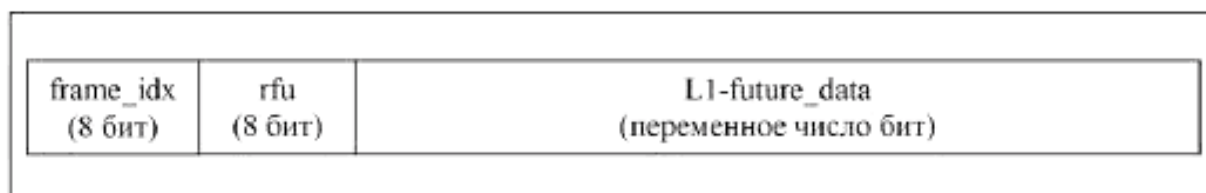
Рисунок 7 — Предстоящие L1-данные как полезная нагрузка
