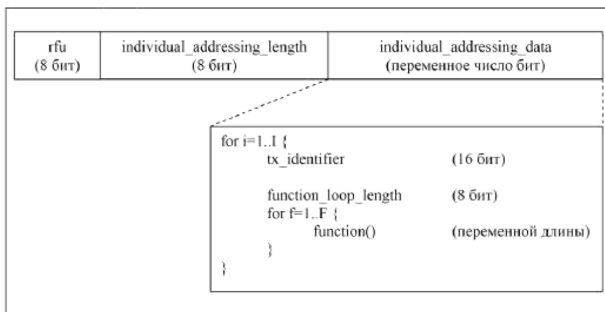
Рисунок 10 — Индивидуальная адресация как полезная нагрузка
