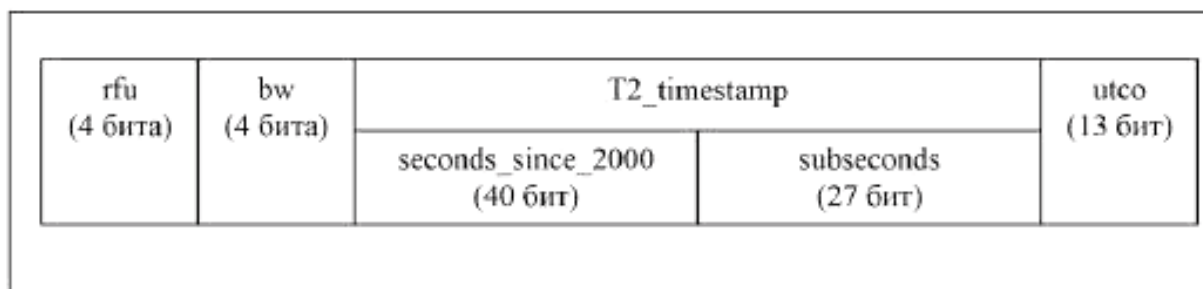
Рисунок 9 — Временной штамп DVB-T2 как полезная нагрузка
