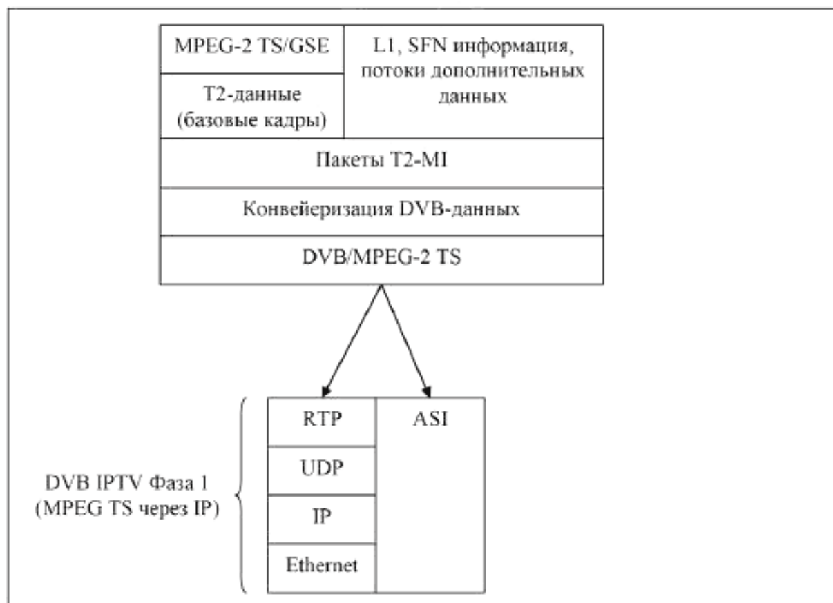
Рисунок 1 — Стек протоколов T2-MI
