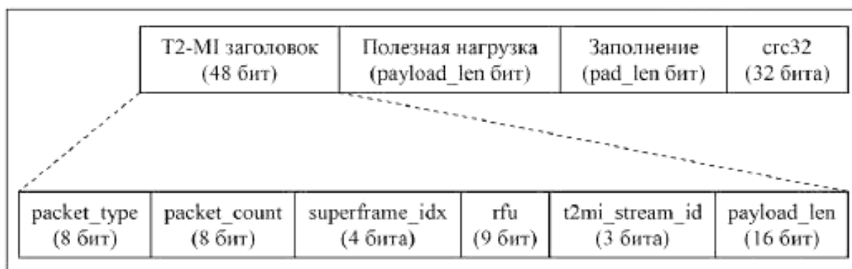
Рисунок 2 — Формат пакета T2-MI
