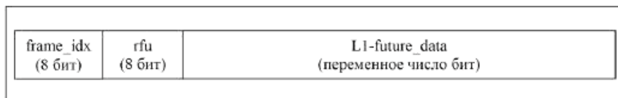
Рисунок 8 — Ячейки балансировки смещения P2 как полезная нагрузка
