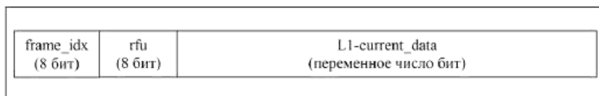
Рисунок 6 — Текущие L1-данные как полезная нагрузка
