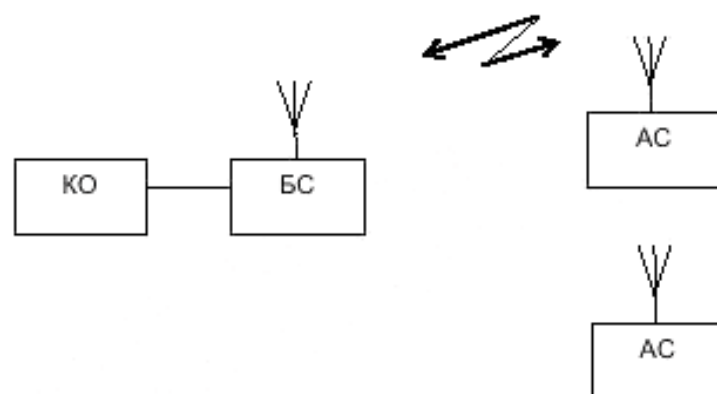
Рисунок 4.1 — Структурная схема организации однозоновой сети подвижной радиосвязи
