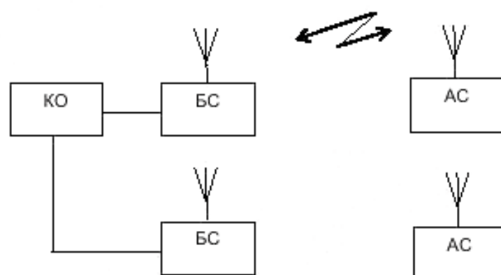
Рисунок 4.2 — Структурная схема организации многозоновой сети подвижной радиосвязи
