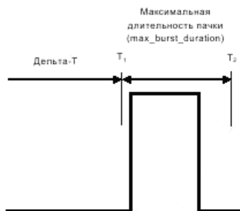
Р и с у н о к 7 — Максимальная длительность пачки
