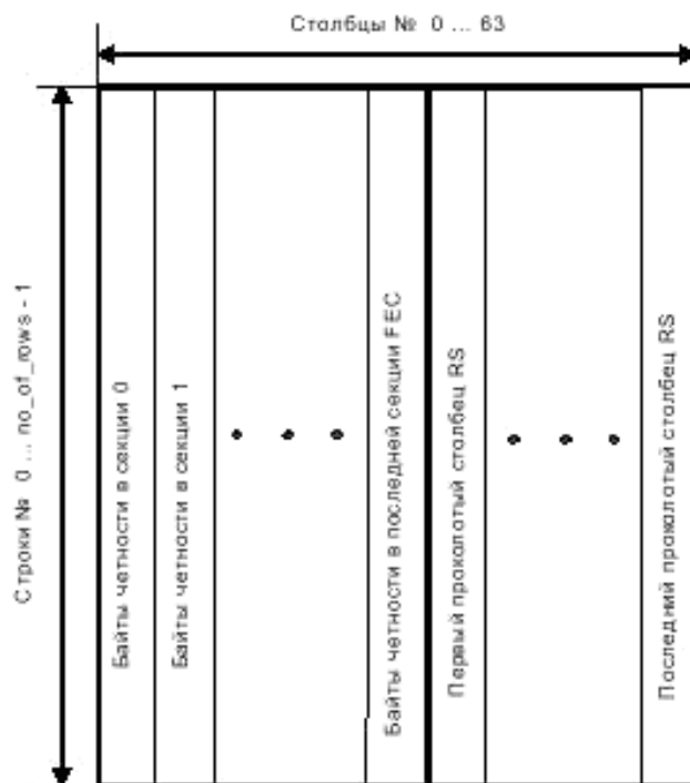
Р и с у н о к 11 — Схема таблицы данных Рида-Соломона
