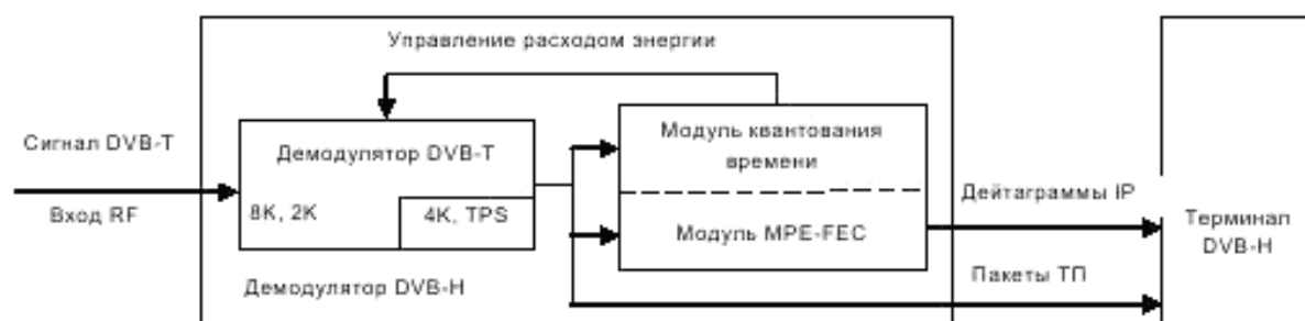
Р и с у н о к 1 — Концептуальная структура приемника DVB-H
