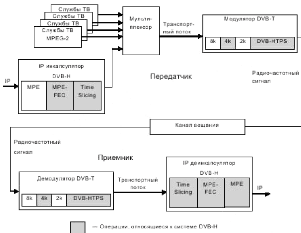
Р и с у н о к 3 — Структура системы DVB-H
