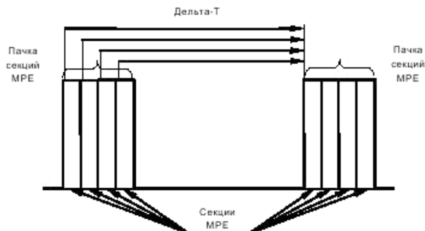
Р и с у н о к 2 — Диаграмма передачи секций MPE в пачках
