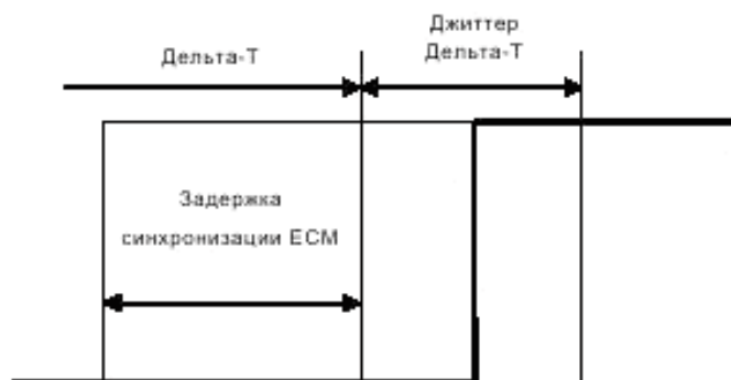
Рисунок 5 — Временная диаграмма джиттера Дельта-Т Figure 6:
