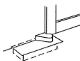
д) Скрытый доводчик нижнего расположения, монтируемый в пол (тип ДП)
