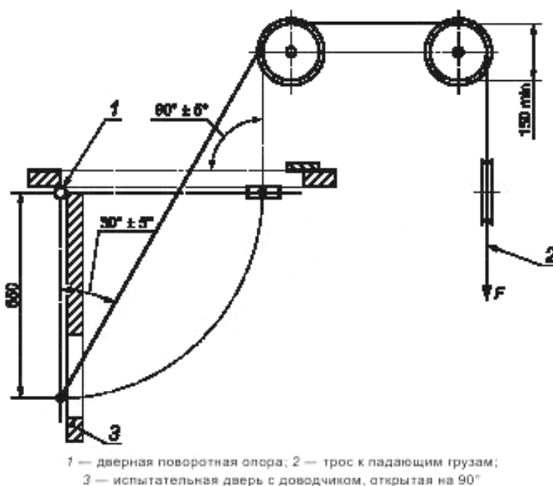
Рисунок Д.4 — Приспособление для испытания доводчиков с перегрузкой
