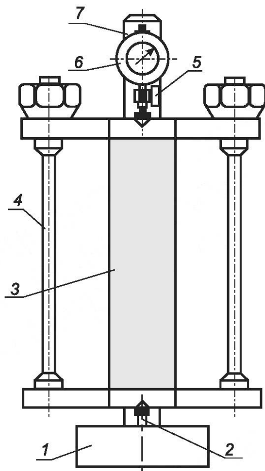
1 — основание измерительного штатива; 2 — шпилька с шаровым наконечником; 3 — образец-балочка; 4 — кондуктор с образцом; 5 — винт крепления индикатора; 6 — индикатор; 7 — стойка измерительного штатива
