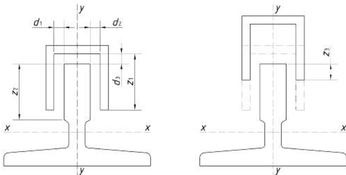
а) Номинальное положение и зазоры контрольного башмака
