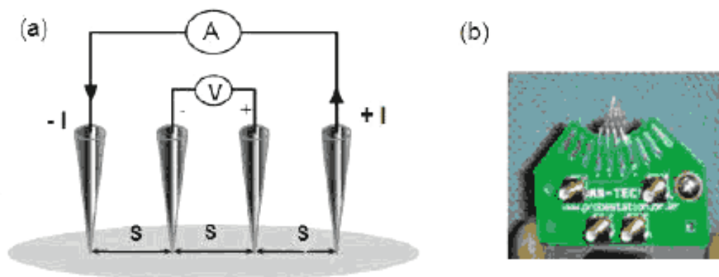
(а) Схема измерительной установки: S — расстояние между зондами; A — источник постоянного тока; V — прибор для измерения электрического напряжения. (б) Фотография измерительной четырехзондовой головки.
