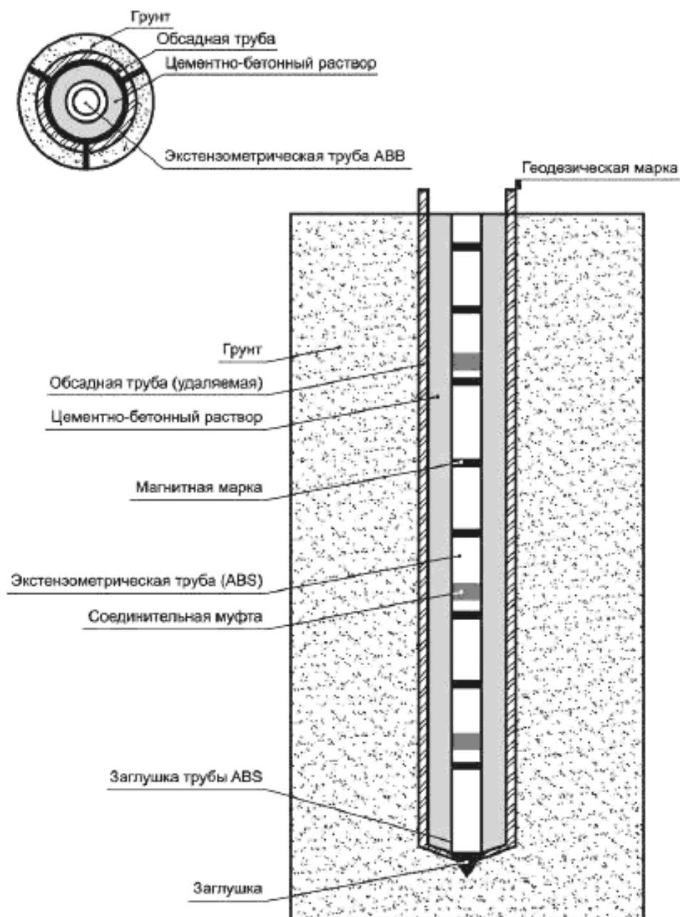
Рисунок Д.2 — Схема экстензометрической наблюдательной скважины
