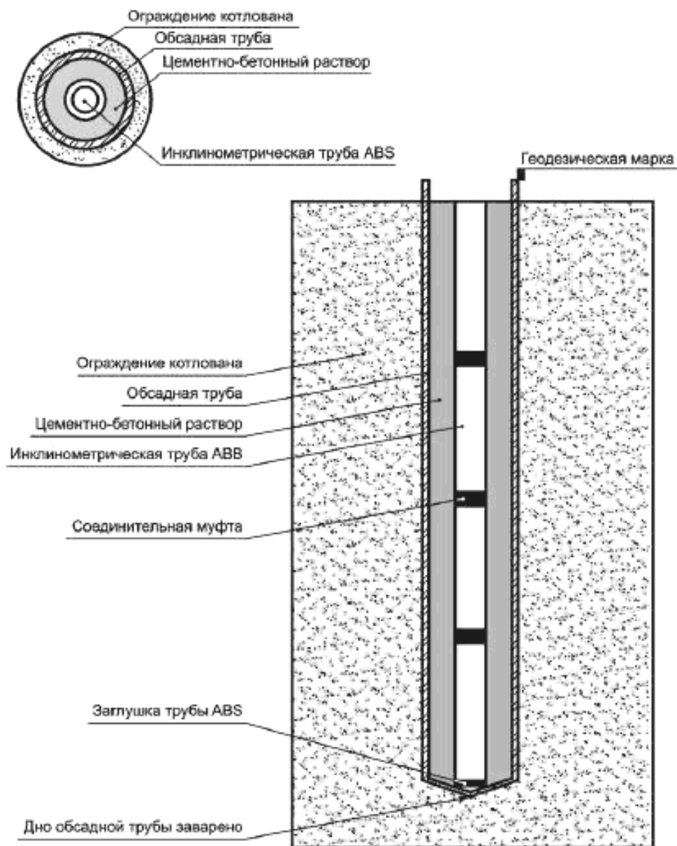
Рисунок Д.1 — Схема инклинометрической наблюдательной скважины
