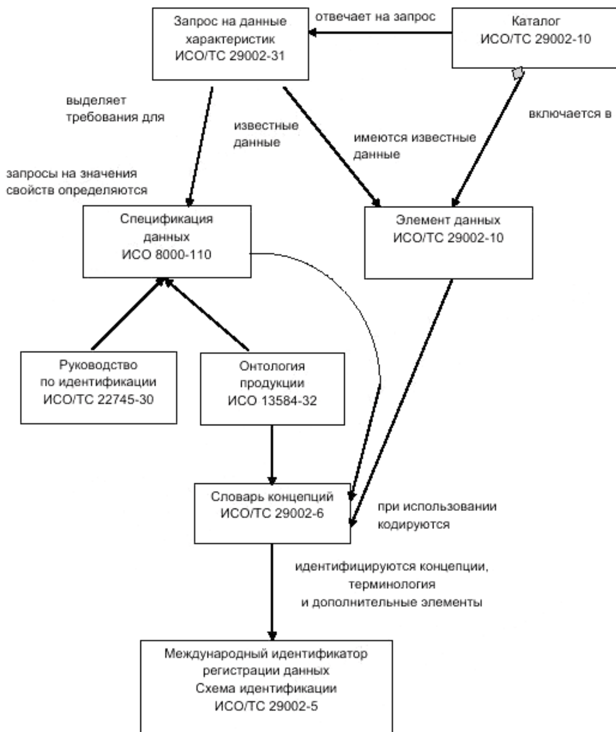
Р и с у н о к 1 — Модель планирования высокого уровня
