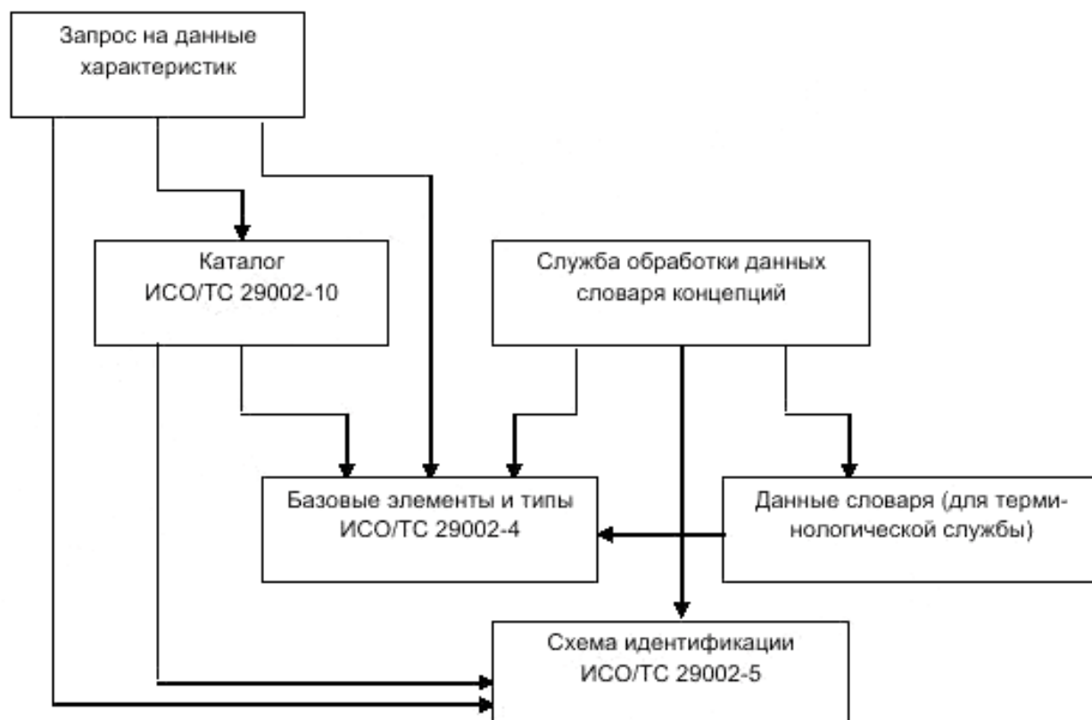
Р и с у н о к 2 — Диаграмма зависимости частей и уровней
