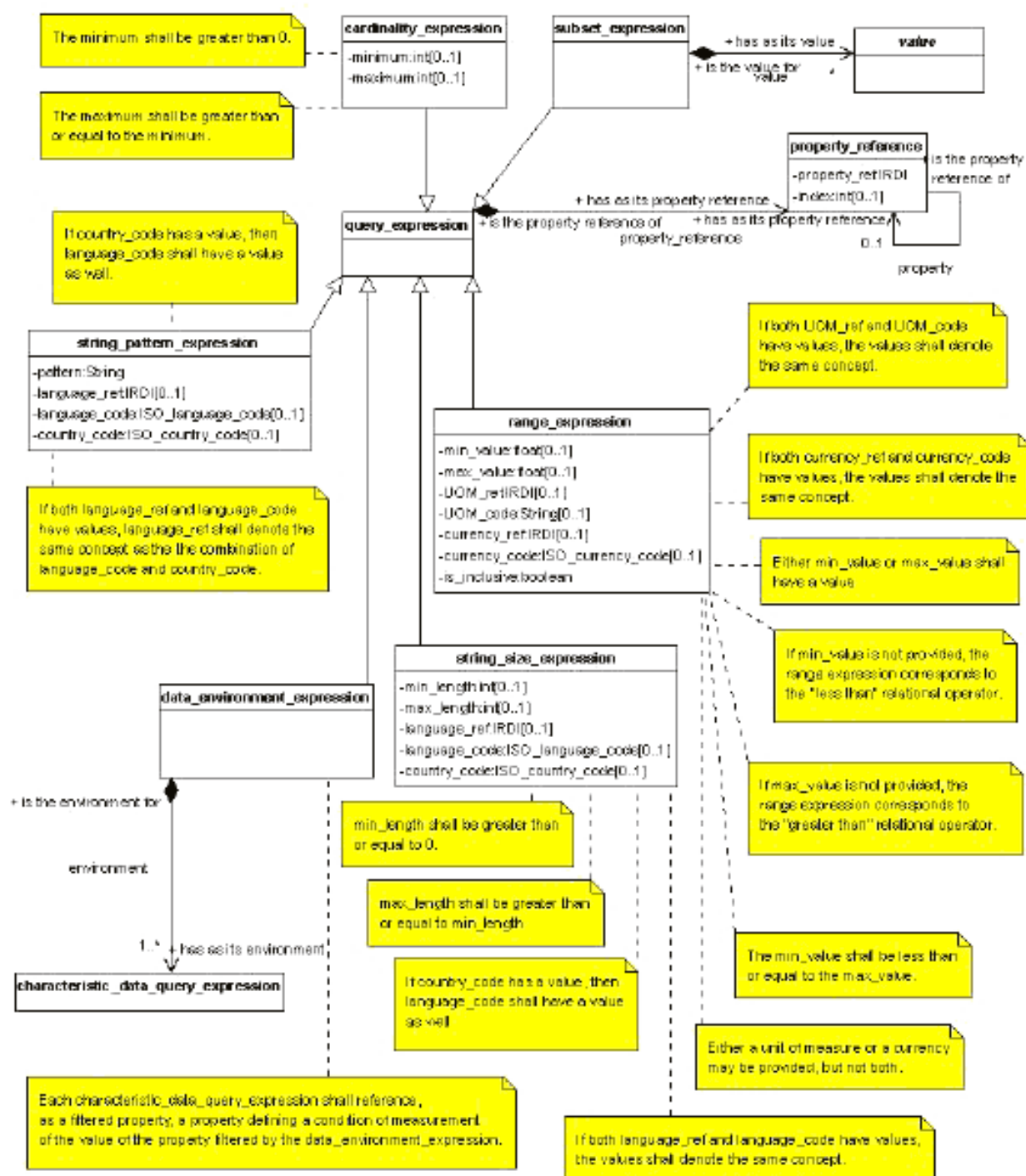
Р и с у н о к 5 — Диаграмма класса UML для формулировки запроса
