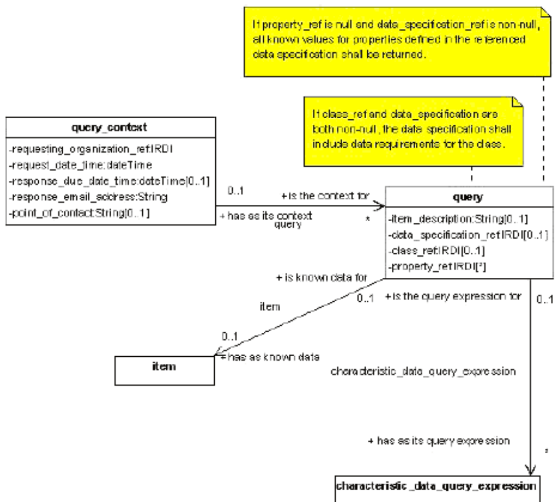
Р и с у н о к 4 — Диаграмма класса UML для основного запроса
