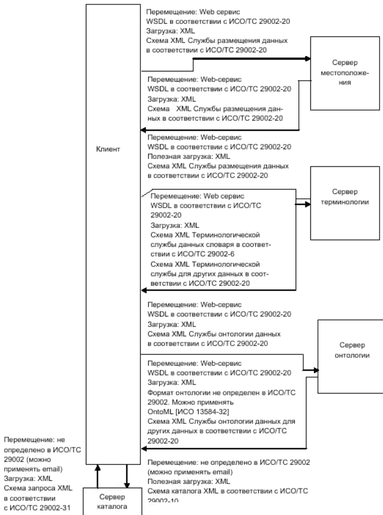
Р и с у н о к 3 — Главные информационные потоки
