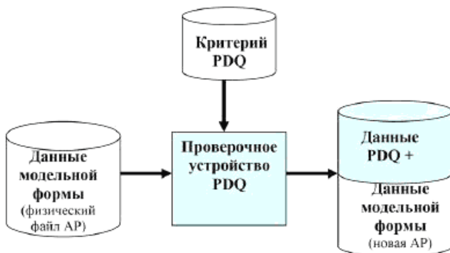
Рисунок 5 — Подход к модификации существующих APs для соответствия их с PDQ-S
