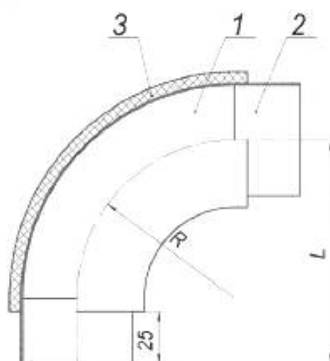
Рисунок А.1 – Конструкция предварительно изолированной стальной трубы
