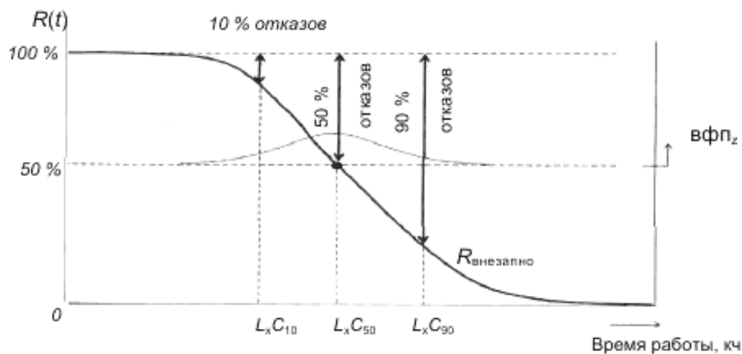
Рисунок С.4 – Кривая надежности внезапного прекращения свечения R_{\text{внезапно}}
