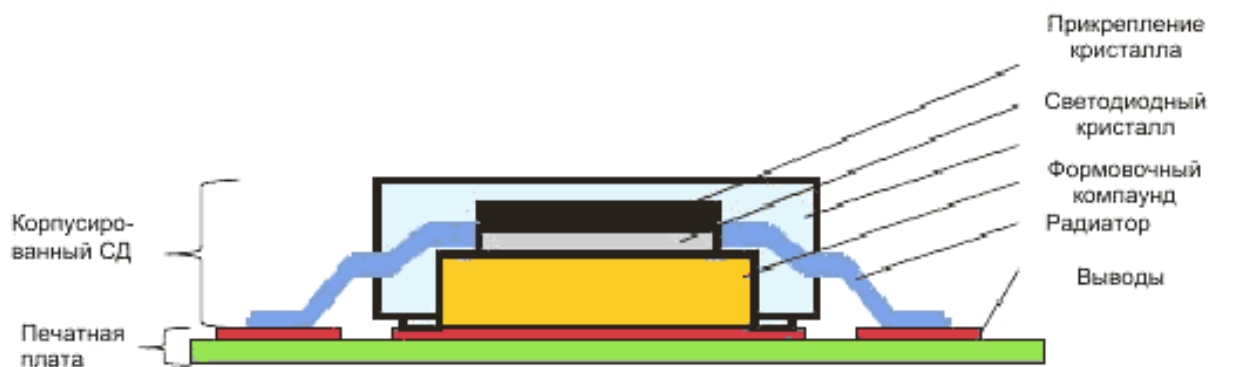
а) Поверхностный монтаж корпусированного СД с выводами
