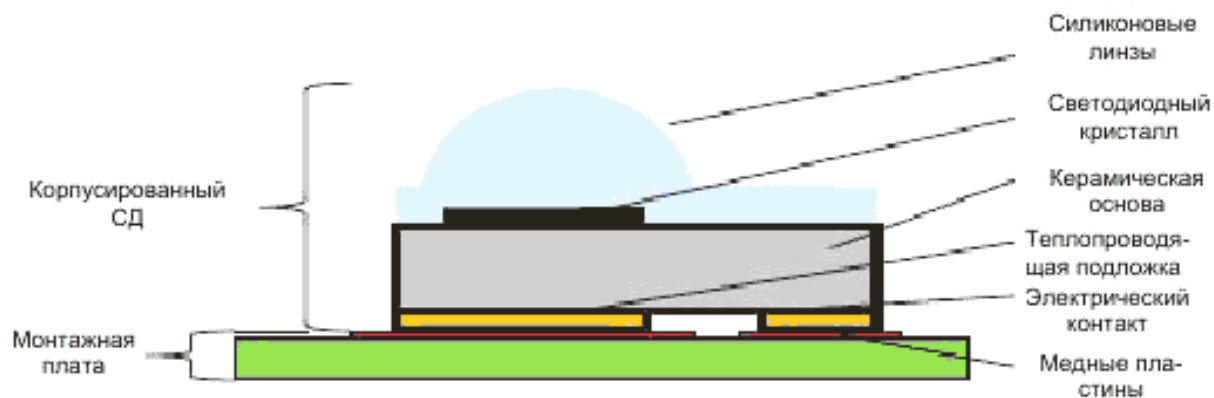
б) Поверхностный монтаж корпусированного СД без выводов
