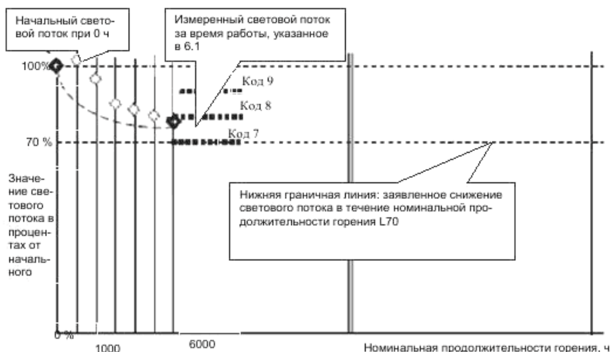
Рисунок 2 – Снижение светового потока в течение времени испытания
