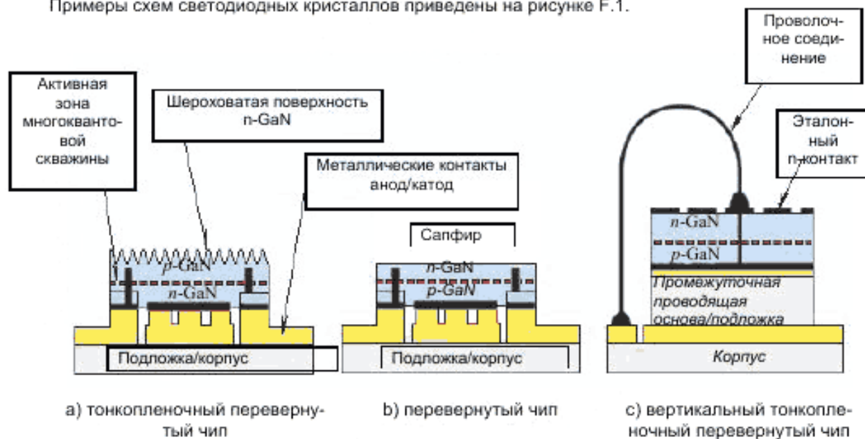
Рисунок F.1 – Схемы светодиодных кристаллов
