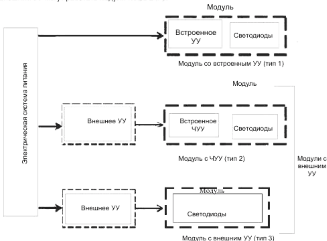
Рисунок 1 – Типы светодиодных модулей
