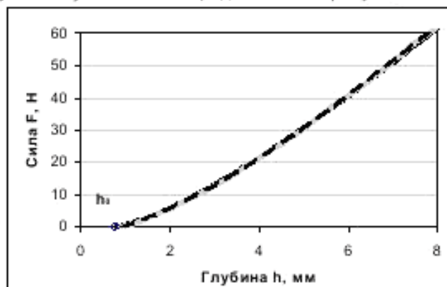
Рисунок 4 – Нахождение нулевой точки h_0
