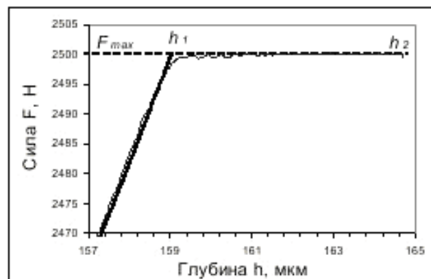
Рисунок 5 – Пример аппроксимации верхней части кривой нагрузки
