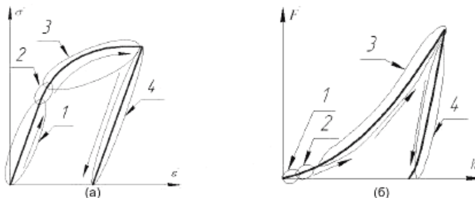
Рисунок Е.1 Схематичное изображение диаграмм: (а)растяжения, (б)вдавливании сферического индентора.
