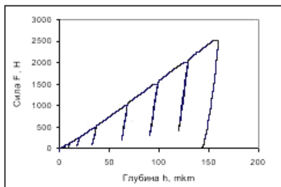
Рисунок 3 – Вид многоциклового диаграммы вдавливания
