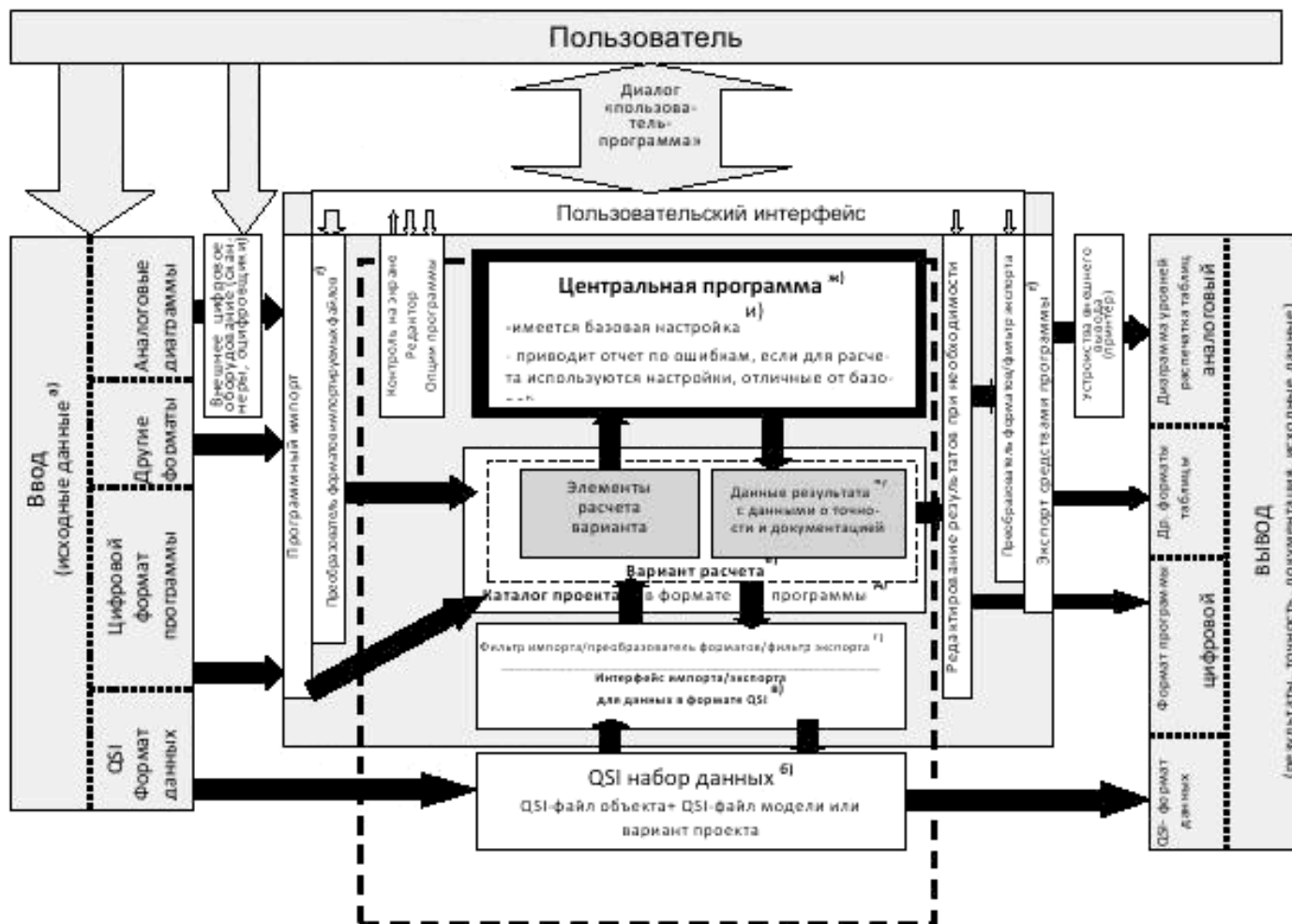
Рисунок Д.1 – Блок-схема потока данных
