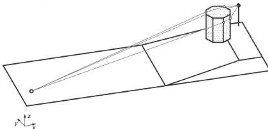
Рисунок 24 — Трехмерное изображение для сценария T14
