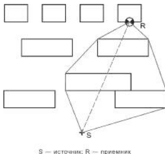
Рисунок 3 — Две расчетные траектории в плоскости EL
