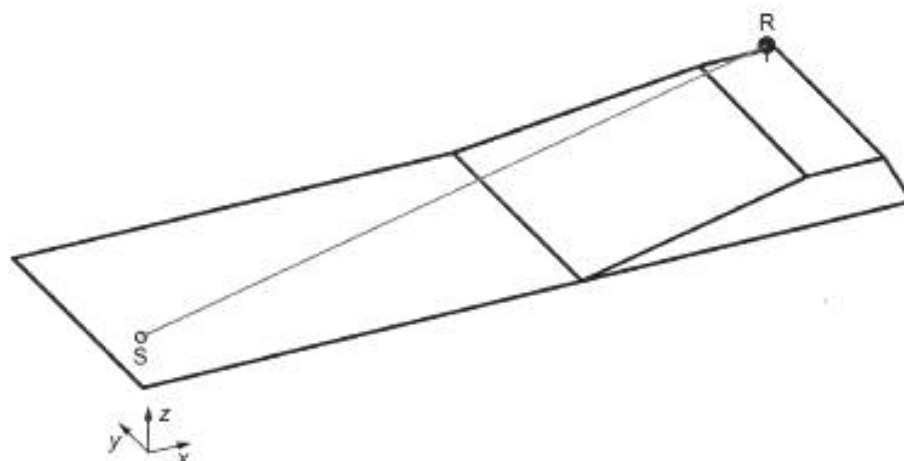
Рисунок 10 — Трехмерное изображение для сценария T06
