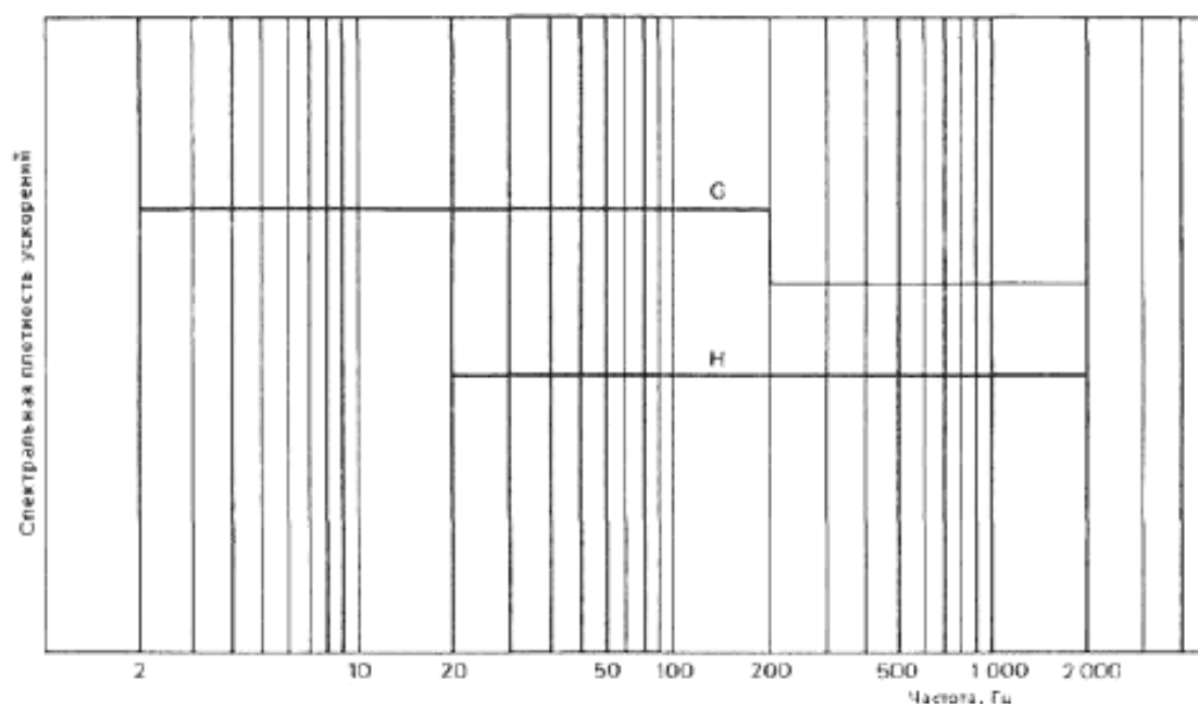
Рисунок 2 — Спектр модели под действием случайной вибрации
