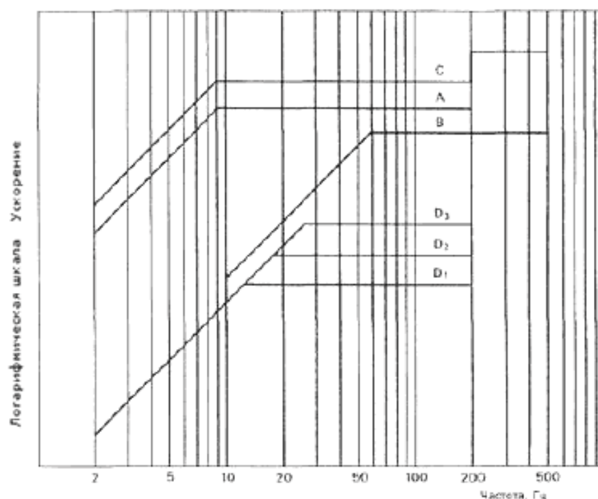
Рисунок 1 — Спектр модели под действием синусоидальной вибрации
