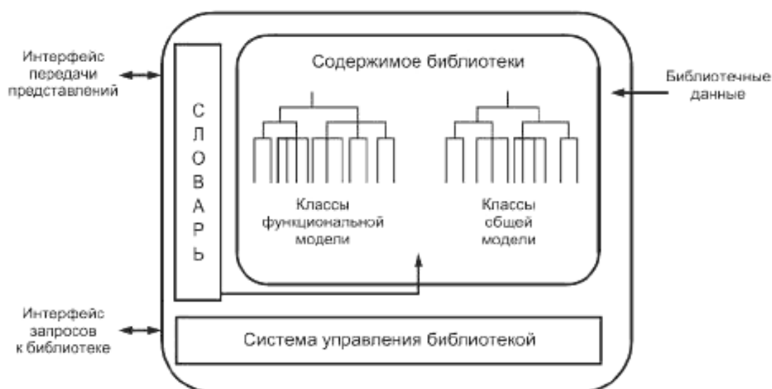
Рисунок 2 — Библиотечная система
