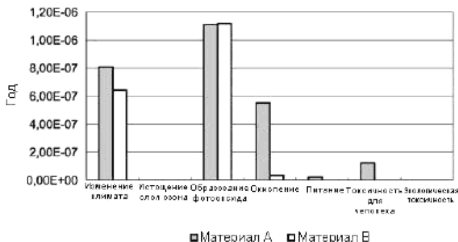
Рисунок 10 — Нормализованный профиль ОВЖЦ для газораспределительной системы
