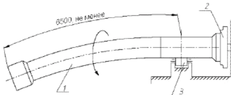
1 – образец с установленными торцевыми заглушками; 2 – патрон токарного станка; 3 – вращающиеся ролики люнетного устройства
