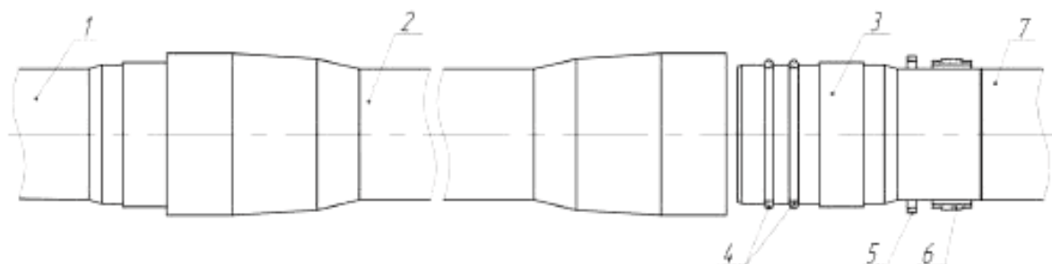
Рисунок 4 – Схема фланцевого соединения труб и фитингов со стальными фитингами и переходными деталями нефтепроводов
