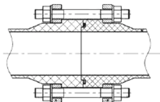
Рисунок А.6 – Вариант фланцевого соединения труб
