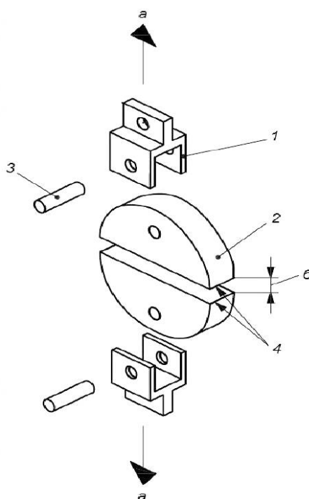
1 – вильчатый захват; 2 – поверхность полудиска, на которую устанавливают образец; 3 – фиксирующий штифт; 4 – закругленные кромки полудисков; а – направление приложения нагрузки; б – расхождение полудисков
