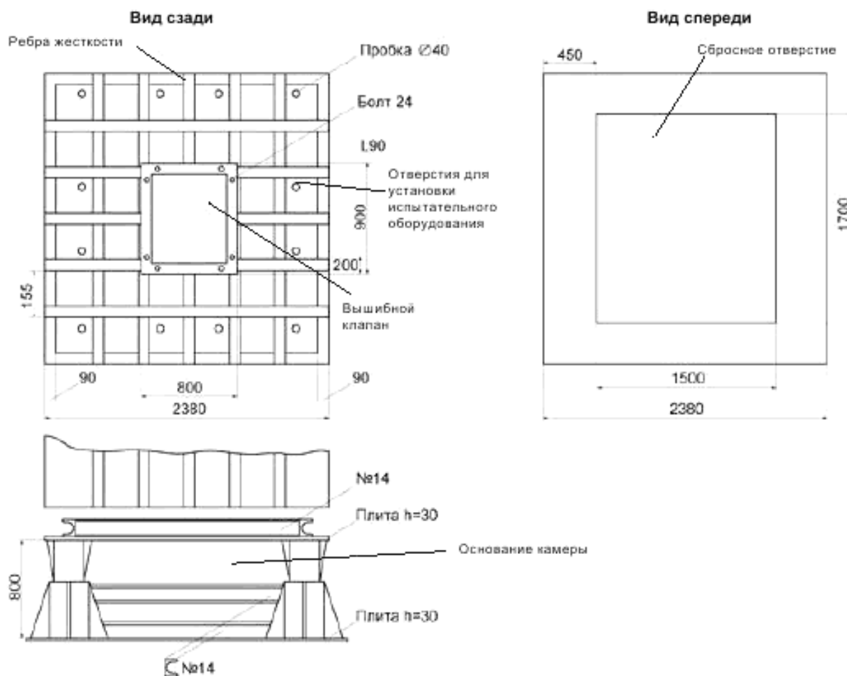
Рисунок А.1 – Схема испытательной взрывной камеры
