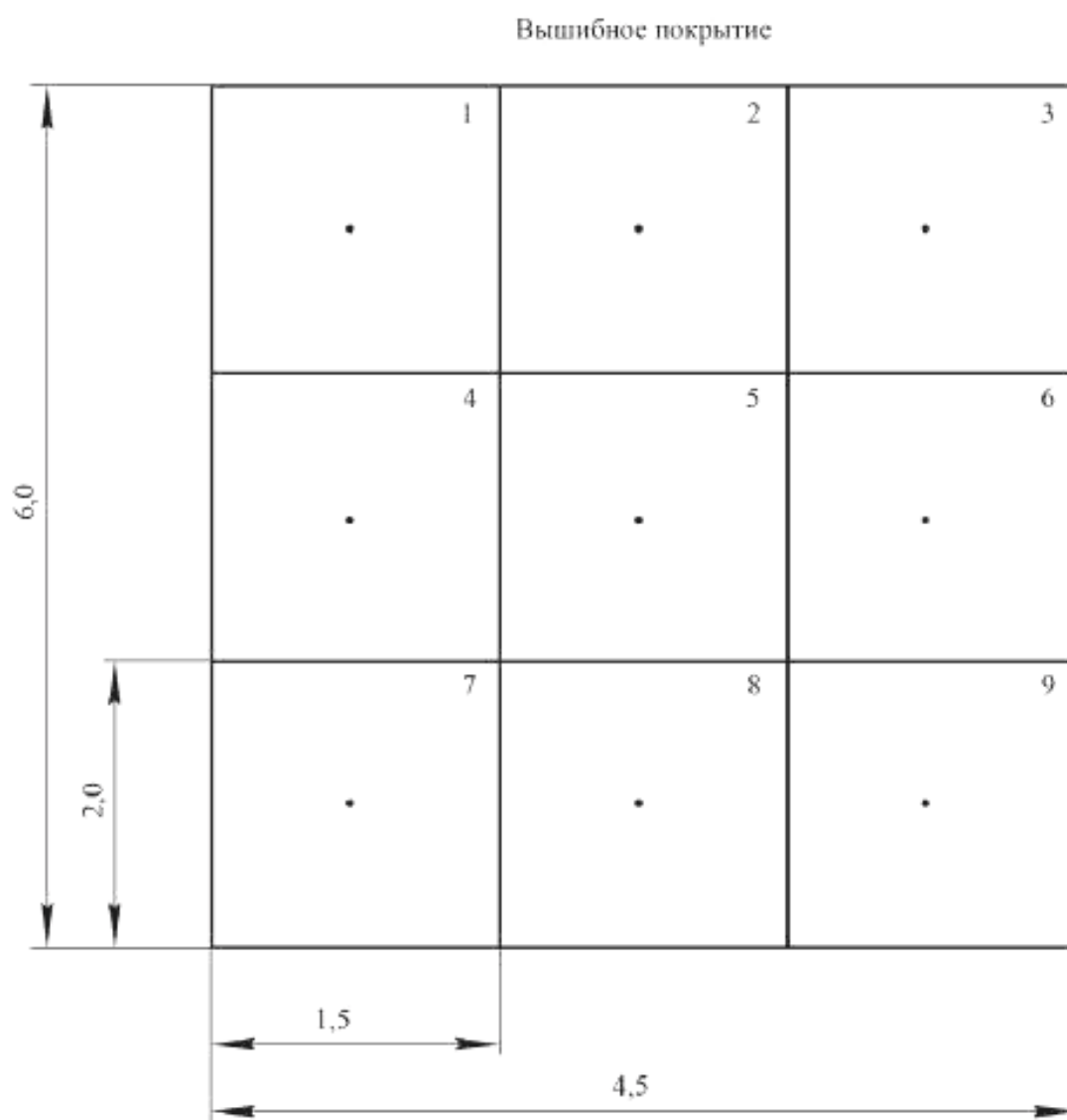
Рисунок А.3 – Схема расположения секторов задней стены
