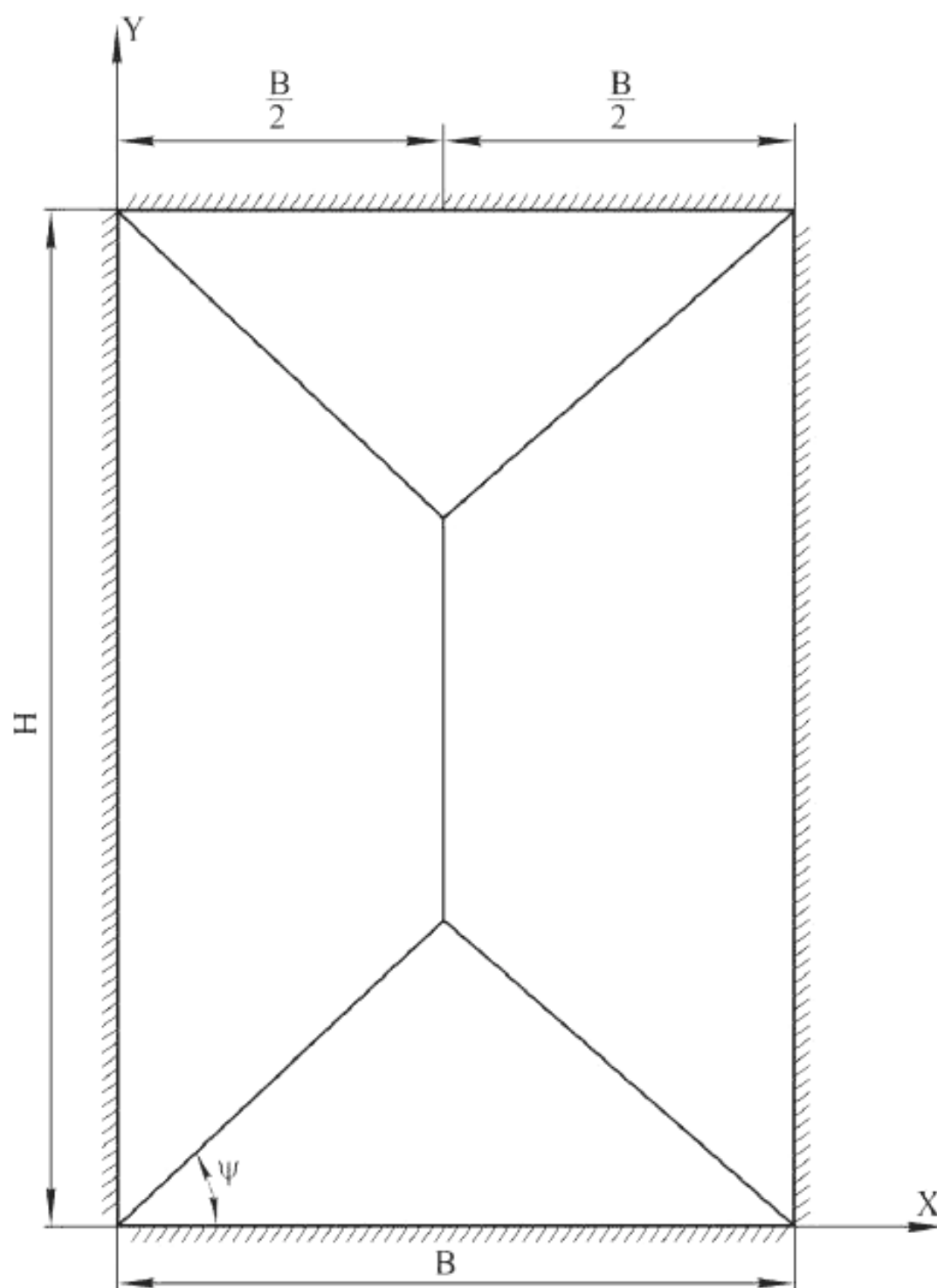
Рисунок 15 – Схема излома задней стены при H > B
