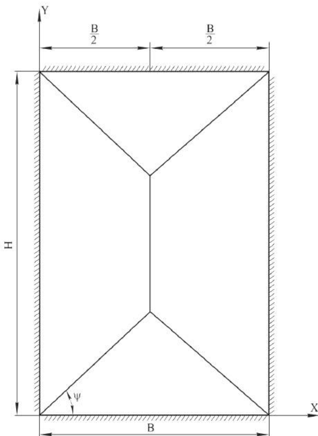
Рисунок 15 – Схема излома задней стены при H > B
