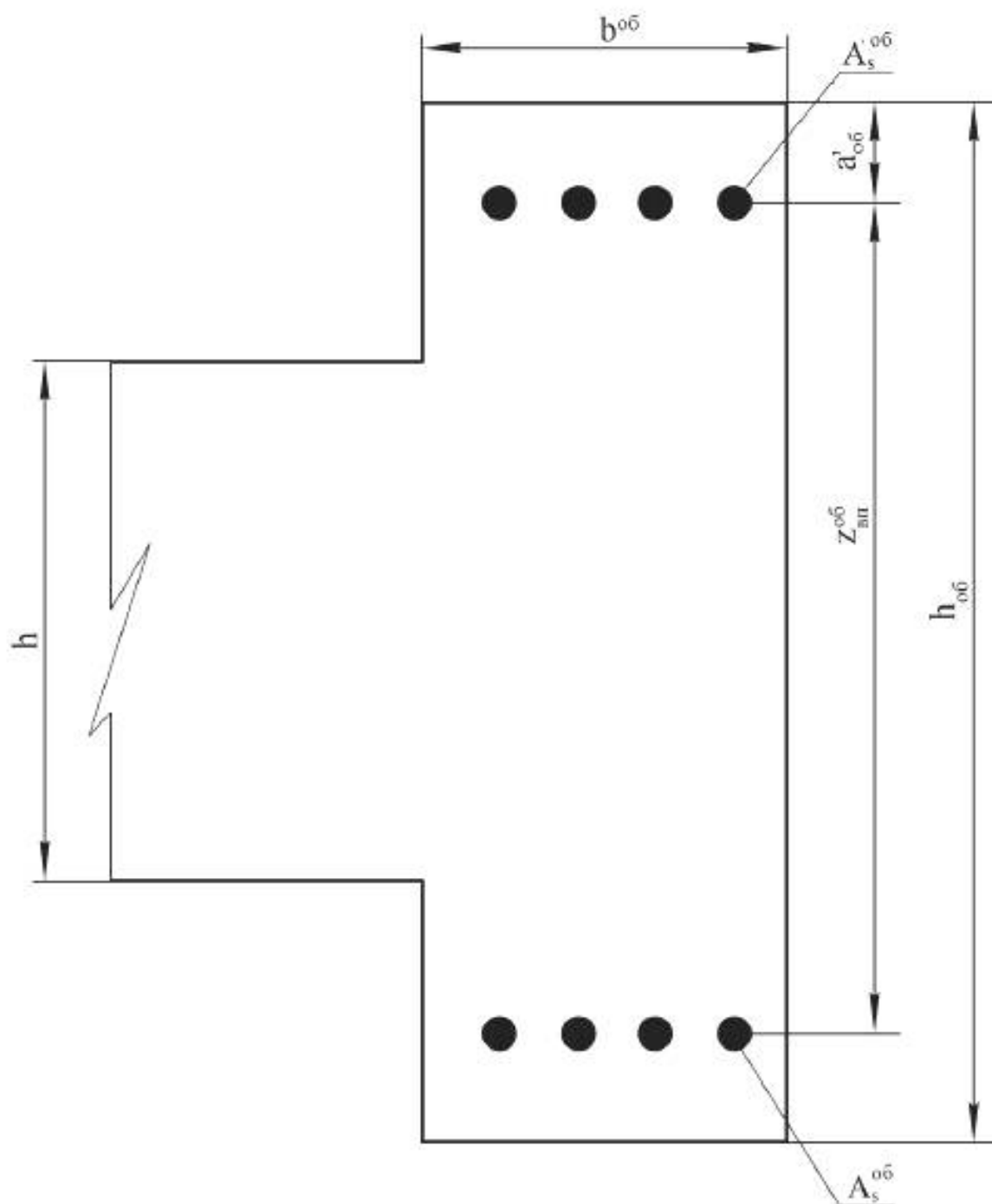
Рисунок 8 – Поперечное сечение обвязки
