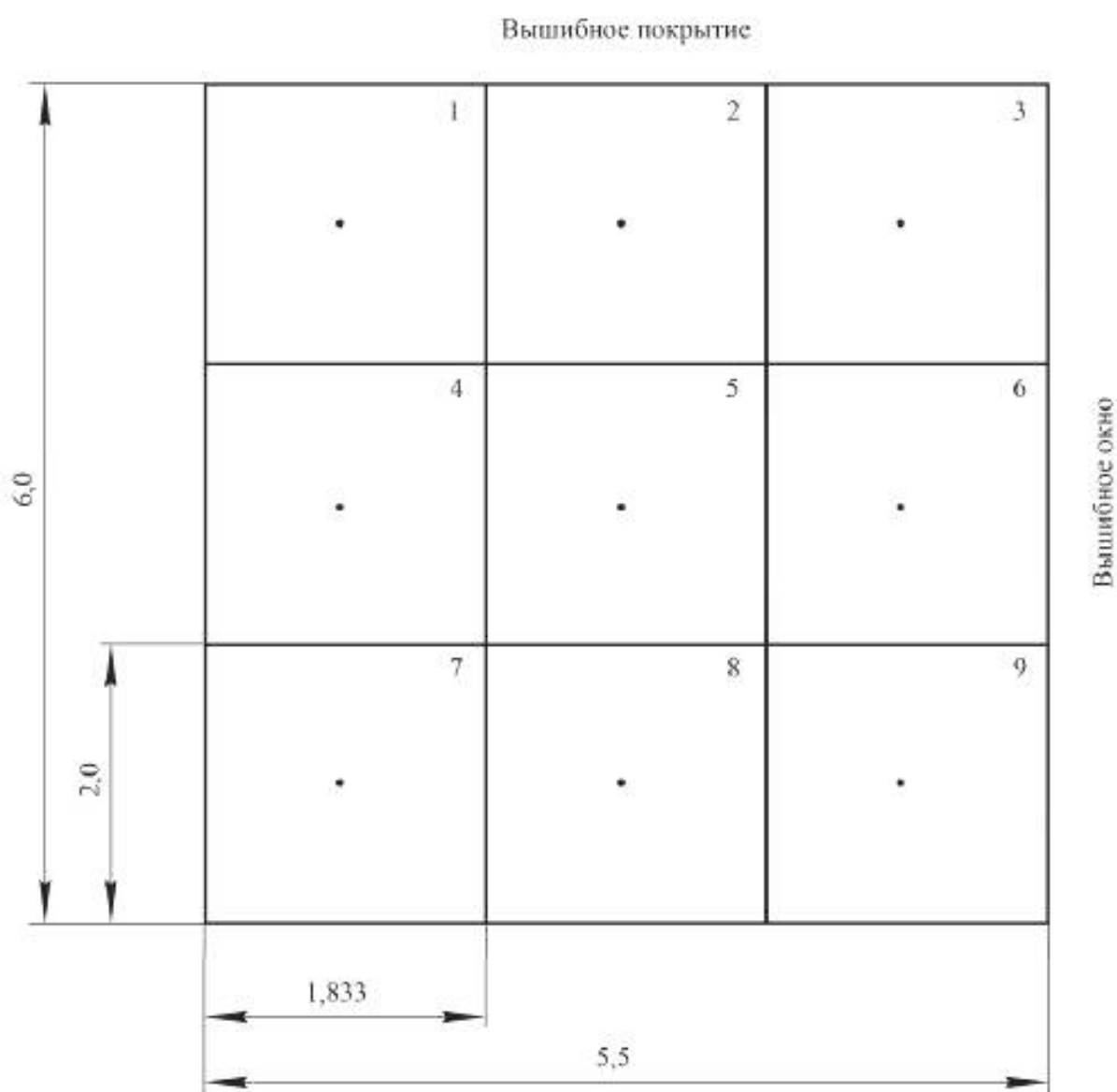
Рисунок А.2 – Схема расположения секторов боковой стены
