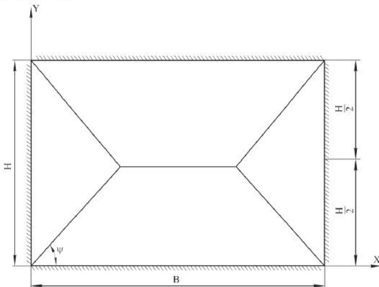
Рисунок 16 – Схема излома задней стены при H < B
