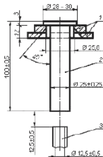
1 – держатель; 2 – образец; 3 – сопло
