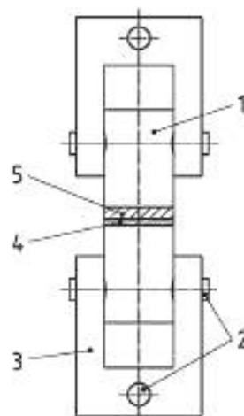
Рисунок 1 – Иллюстрация нагрузочного блока, позволяющего минимизировать внеосевую нагрузку
