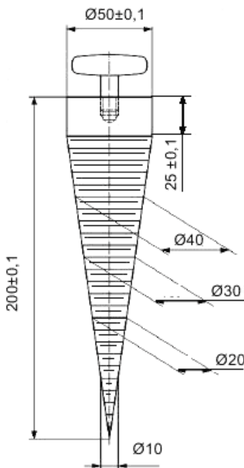
Рисунок 3 – Измерительный конус
