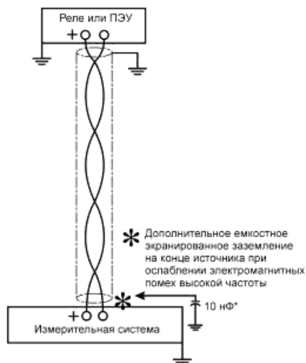
Рисунок 2 — Одна измерительная система и один вход реле
