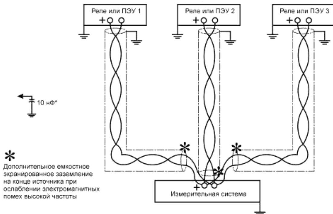
Рисунок 3 — Одна измерительная система с несколькими входами реле
