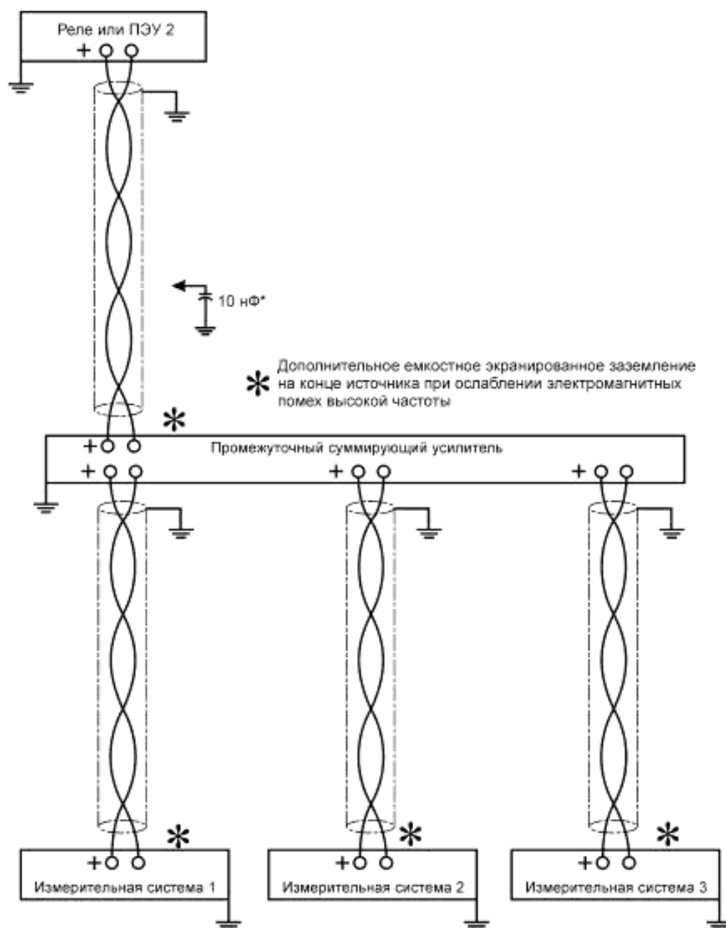
Рисунок 4 — Несколько измерительных систем и промежуточное устройство
