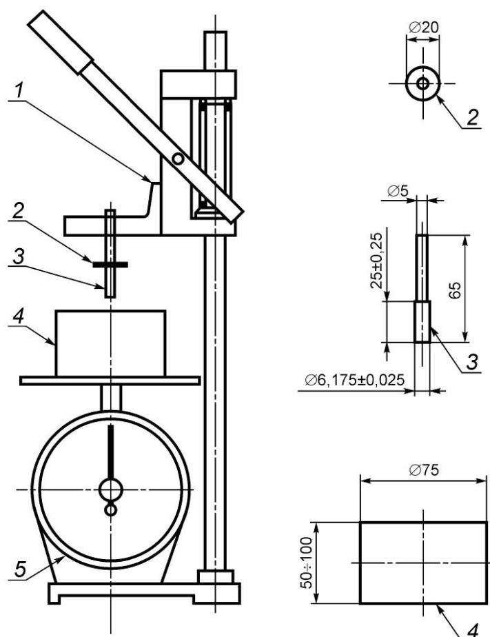
1 — подвижная кулиса со штативом, зажимом и рычажным механизмом, с возможностью перемещения по стойке штатива; ход рычажного механизма не меньше 40 мм; 2 — латунное кольцо; надевается на латунный стержень; 3 — латунный стержень с плоским шлифованным торцом в уширении; 4 — герметичный контейнер для испытуемой ремонтной смеси; 5 — электронные весы с горизонтальной площадкой под контейнер с ремонтной смесью (диапазон взвешивания и шаг взвешивания см. в Б.2.2.5)
