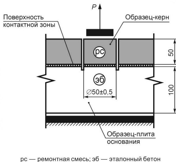
Рисунок Ж.2 — Схема испытаний контрольных образцов с адгезионным соединением контактной зоны на растяжение при отрыве
