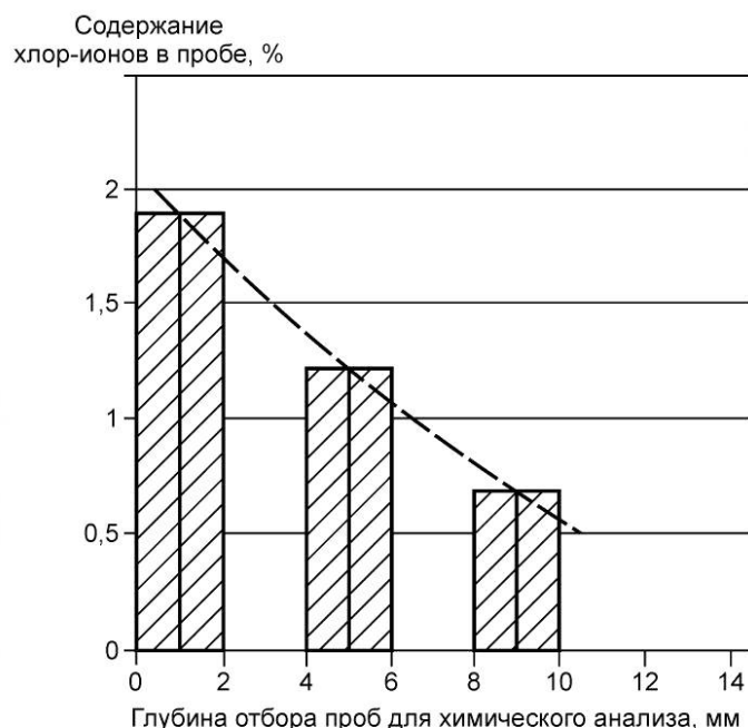
Рисунок Л.2 — Результаты химического анализа проб на содержание хлор-ионов в диапазонах глубины 0—2, 4—6 и 8—10 мм (пример)
