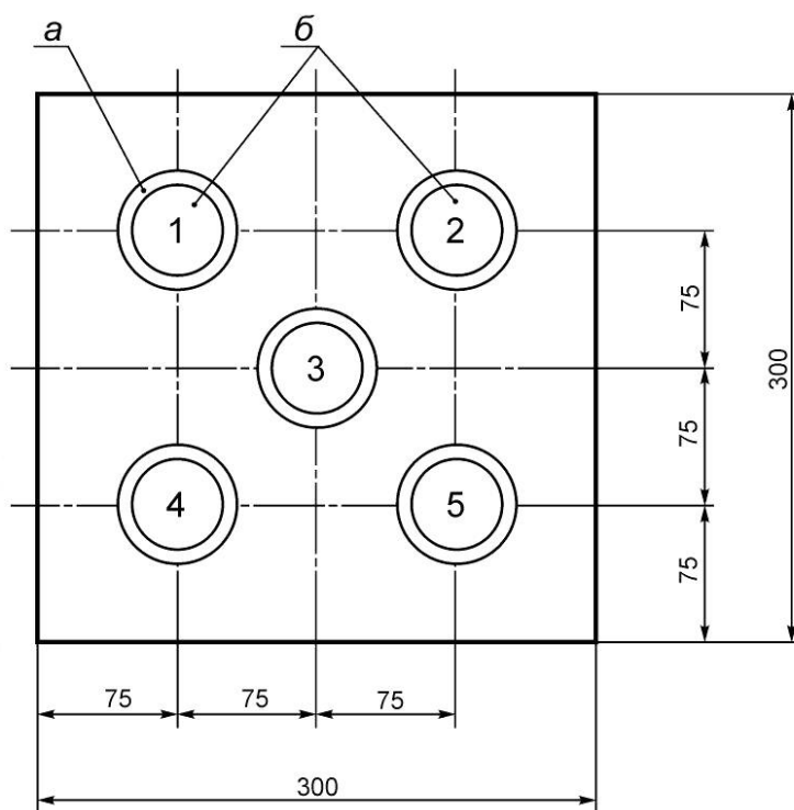
а — цилиндрический пропил; б — образец-кern; 1—5 — маркировка образцов-кernов
