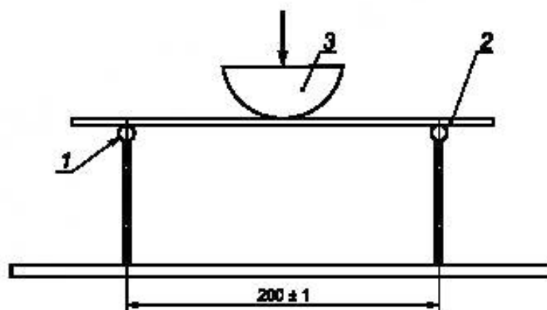
Рисунок Г.4 — Схема проведения испытания
