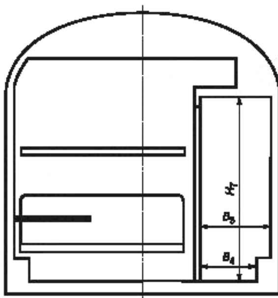
Рисунок 6 — Поперечное сечение кулейного вагона
