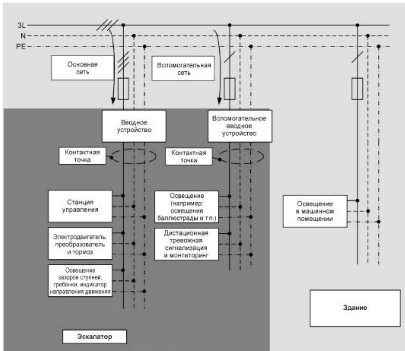
Рисунок А.2 — Подключение средств измерения энергопотребления эскалаторов
