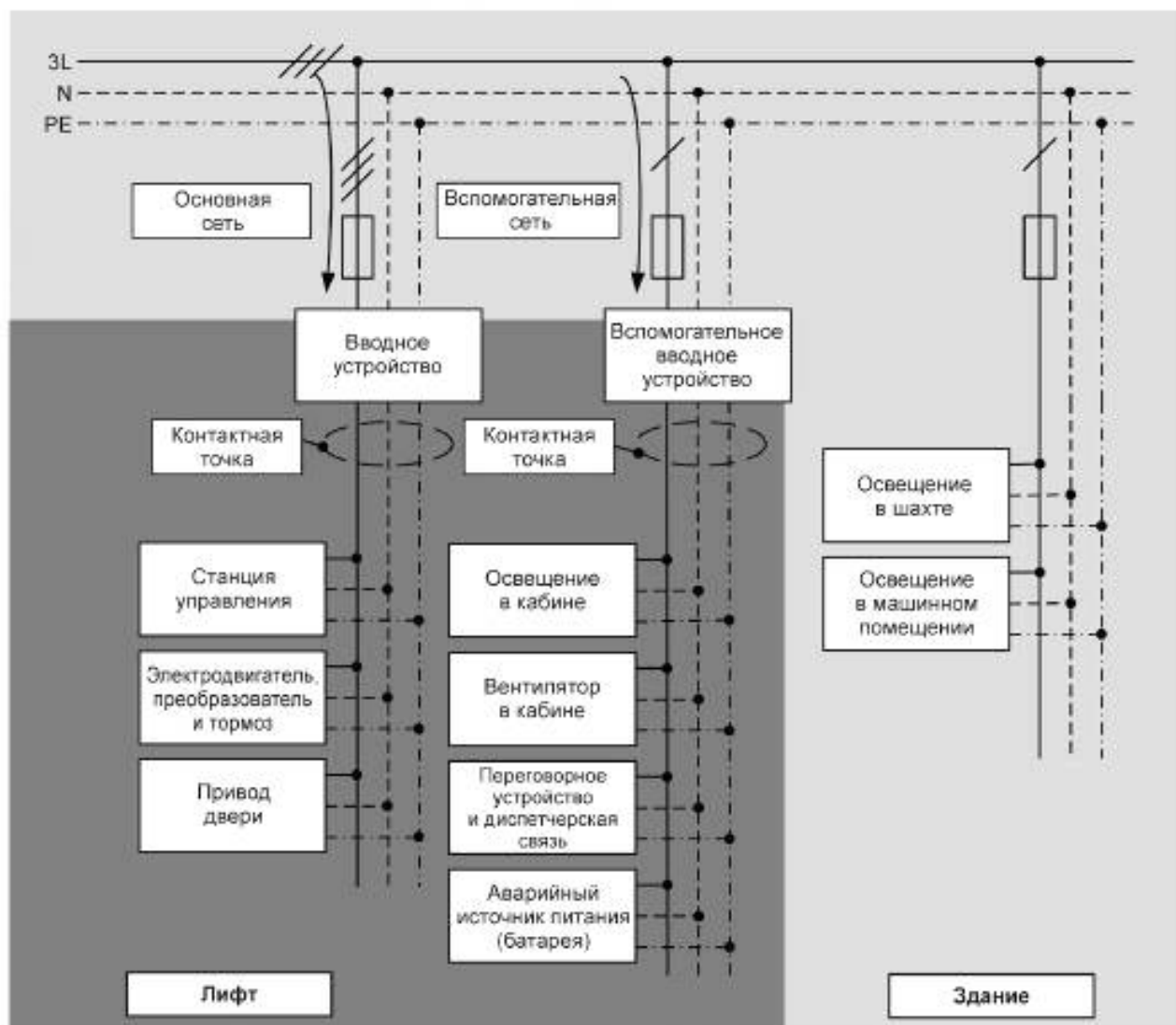
Рисунок А.1 — Подключение средств измерения энергопотребления лифтов
