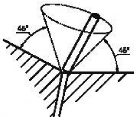
Рисунок Г.3 — Схема вращения стержня-пальца
