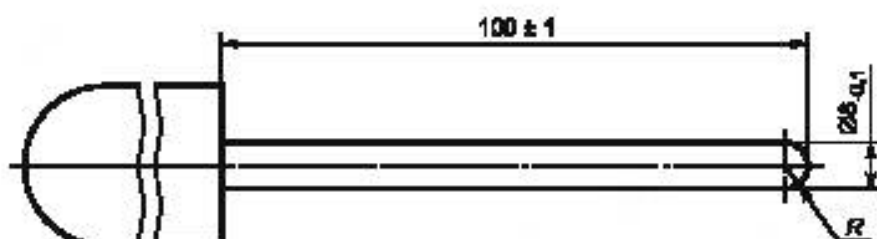
Рисунок Г.1 — Стержень-палец А (малый)
