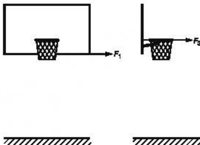
Рисунок Д.3 — Нагружение при испытаниях на прочность
