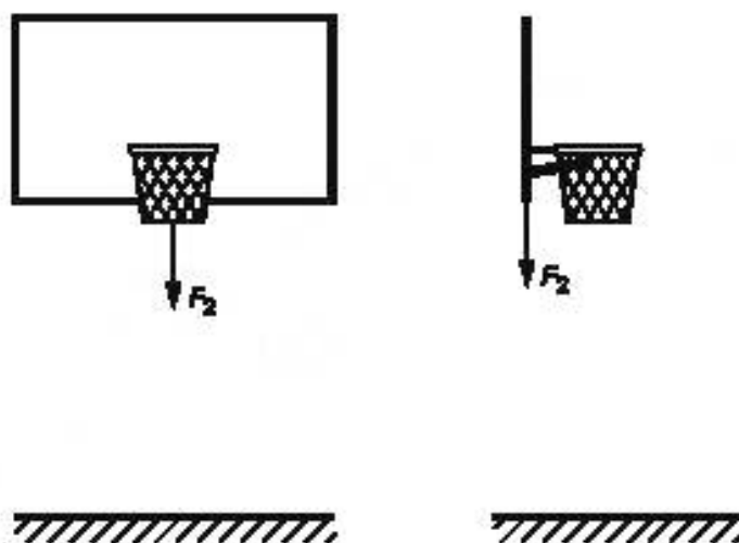
Рисунок Д.4 — Нагружение при испытаниях на устойчивость
