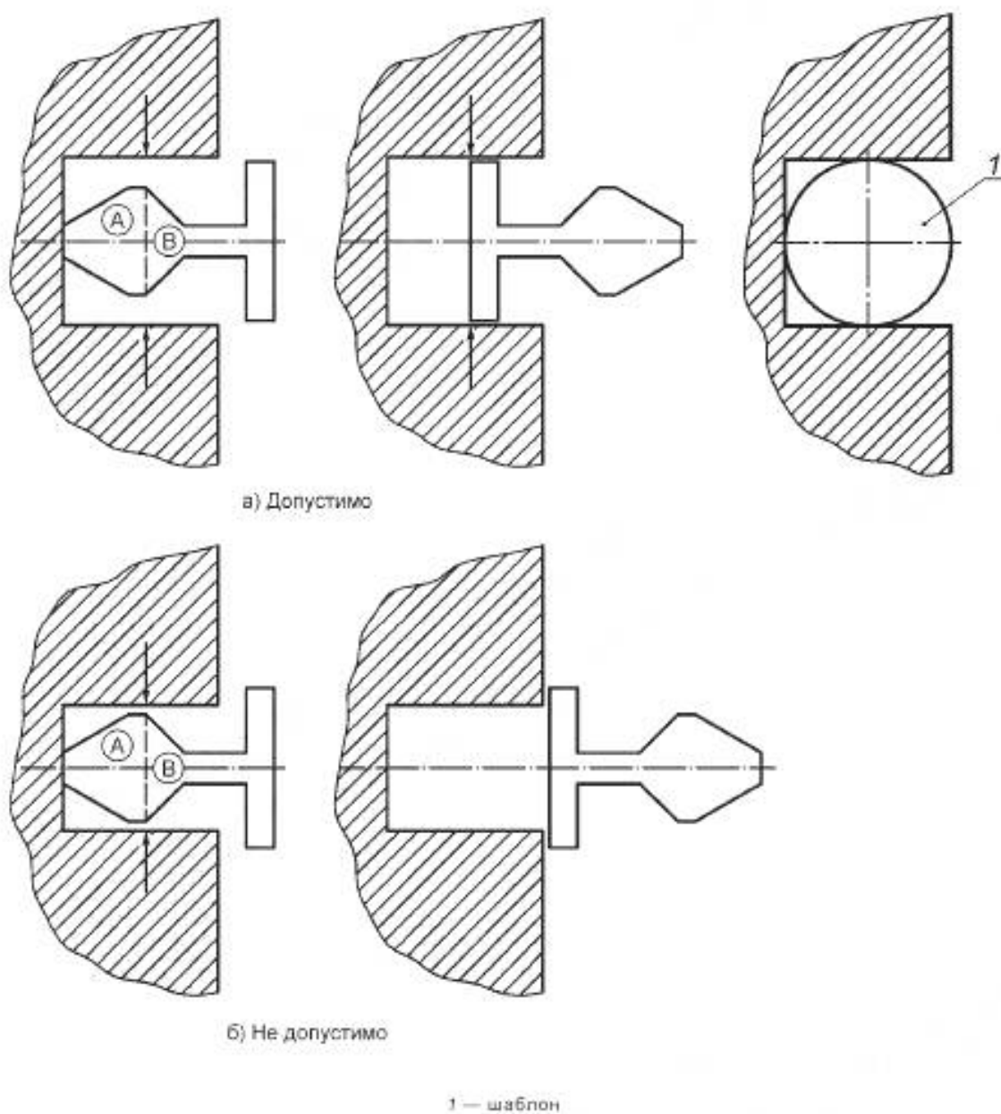
Рисунок Г.11 — Примеры размещения шаблона при испытаниях зазоров, вариант 2
