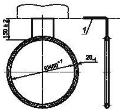
Рисунок 9 — Размеры баскетбольного кольца
