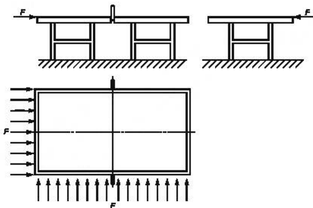
Рисунок Ж.1 — Схема приложения нагрузок при испытаниях
