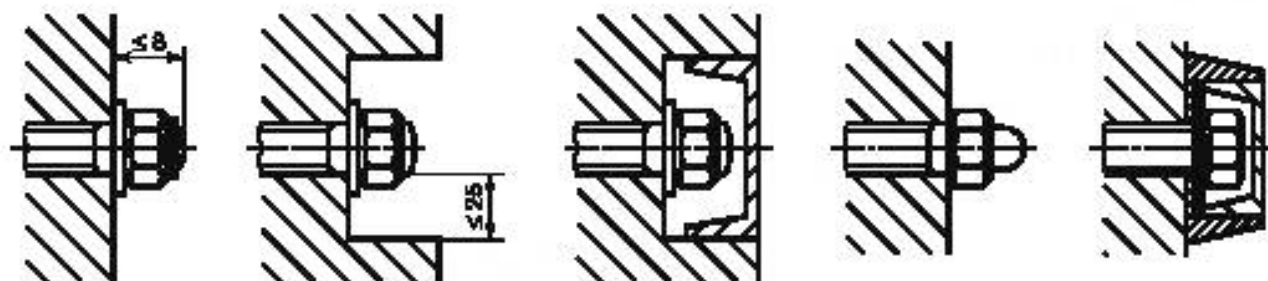
Рисунок 2 — Защита болтовых соединений
