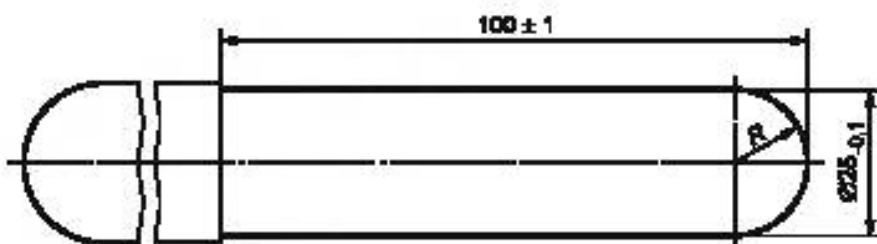
Рисунок Г.1 — Стержень-палец А (малый)
