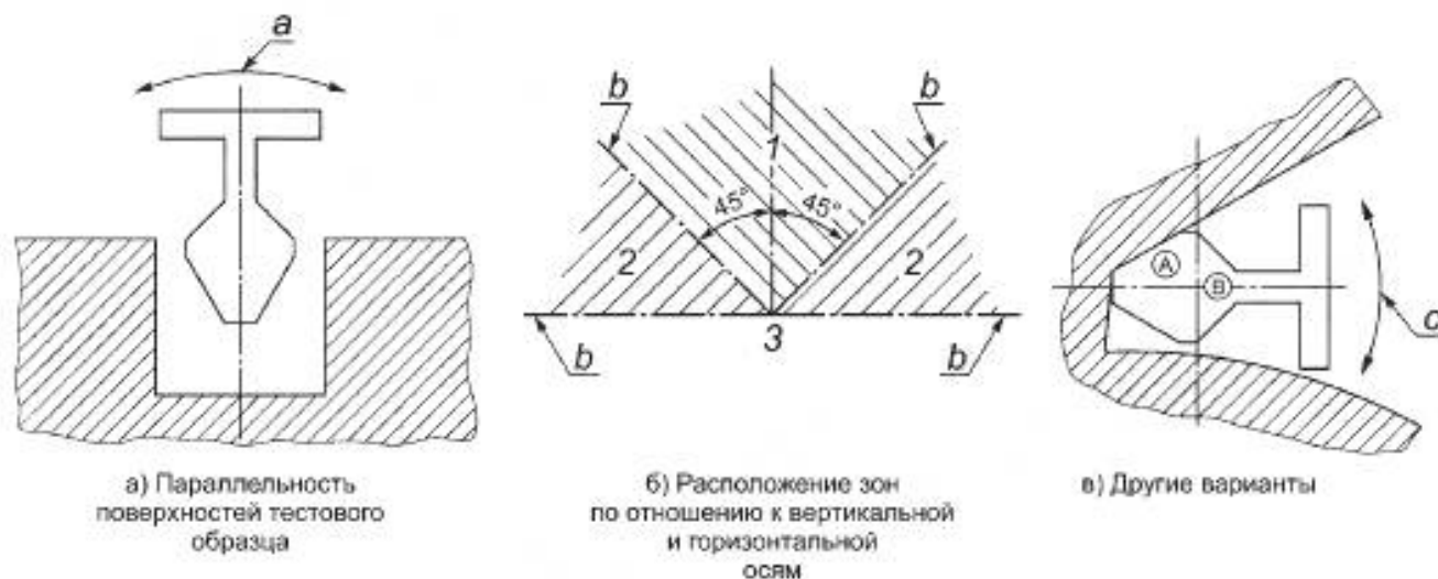
1 — зона 1; 2 — зона 2; 3 — зона 3 а — угол ввода зоны А шаблона; б — ось шаблона; в — проверка всех углов ввода
