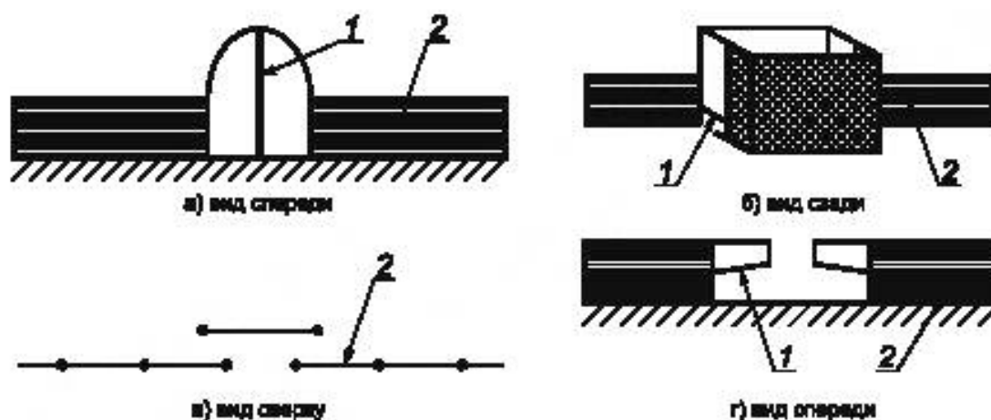
Рисунок 4 — Примеры ожидаемых препятствий
