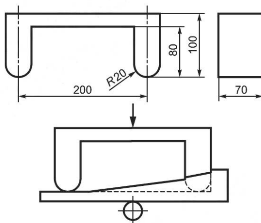
Рисунок 3 — Прибор для испытаний опоры для ступни
