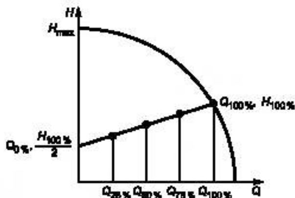
Рисунок 1 — Опорный график производительности циркуляционного насоса
