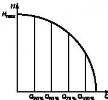
Рисунок 2 — Профиль нагрузки циркуляционного насоса
