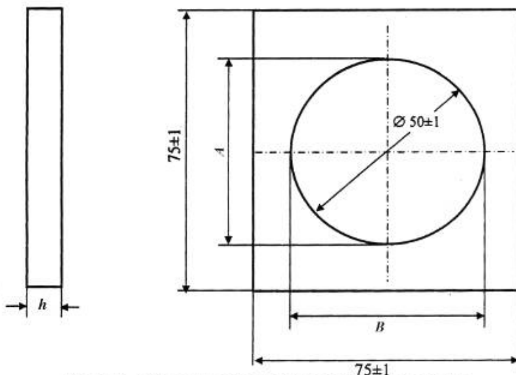
Рисунок 4 – Образец для определения термической релаксации
