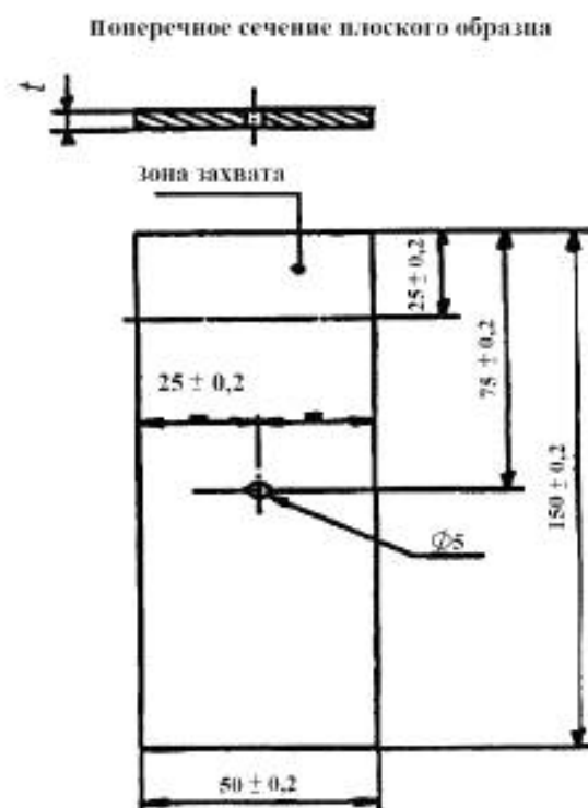
Рисунок 2 – Образец для испытаний на сопротивление распространению трещин
